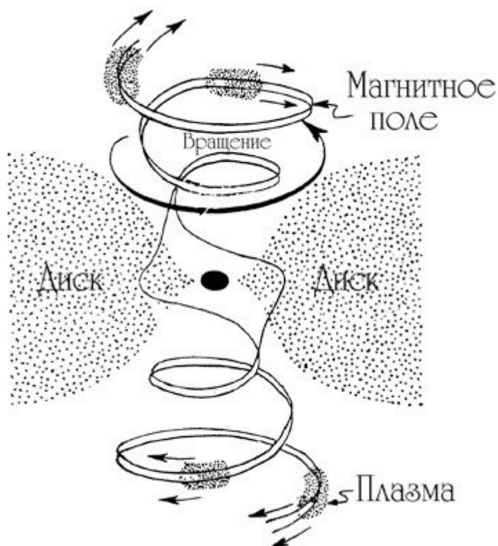
Рис. 9.4. То же, что на рис. 9.3, но магнитное поле привязано к аккреционному диску (Рисунок Мэтта Зимета по моему наброску; из [Торн 2009].)
