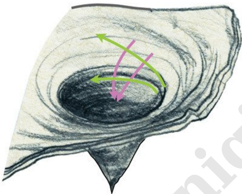
Рис. 4.6. Четыре траектории планетарного движения вблизи черной дыры. Изображение дыры взято с рисунка Лии Хэллоран (рис. 4.5)
