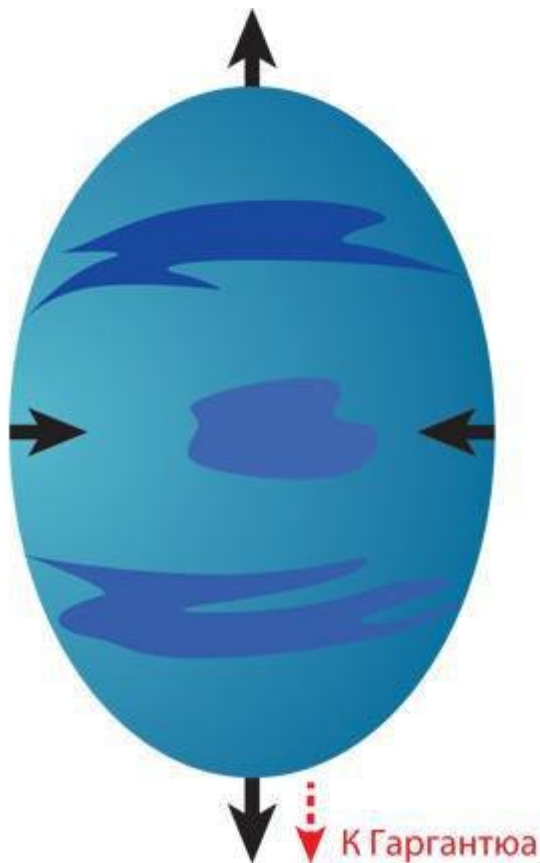
Рис. 6.1. Приливная гравитация Гаргантюа растягивает и сжимает планету Миллер
