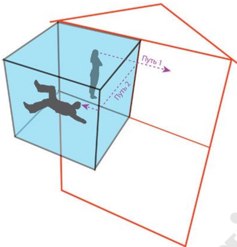
Рис. 29.5. Тессеракт, пристыкованный возле спальни Мёрф
