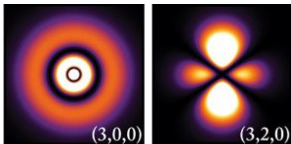
Рис. 26.1. Плотность вероятности местонахождения электрона для двух разных атомов водорода. Вероятность велика для белых областей, меньше для красных и очень мала для черных. (3, 0, 0) и (3, 2, 0) — наборы квантовых чисел, характеризующие эти состояния электрона
