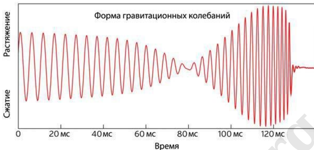
Рис. 16.2. Последние 120 миллисекунд (мс) гравитационных колебаний, зарегистрированных в ЛИГО (График, построенный мной на основе моделирования Янбея Чена, Фукара и других (2011).)
