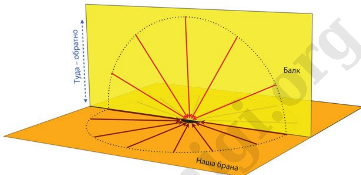
Рис. 23.2. Силовые линии гравитационного поля распространяются в балке радиально, если балк не искривлен. Пунктирные окружности изображены здесь лишь для наглядности (Перерисовка с иллюстрации из книги Лизы Рэндалл «Закрученные пассажи: Проникая в тайны скрытых размерностей пространства» [Рэндалл 2011].)
