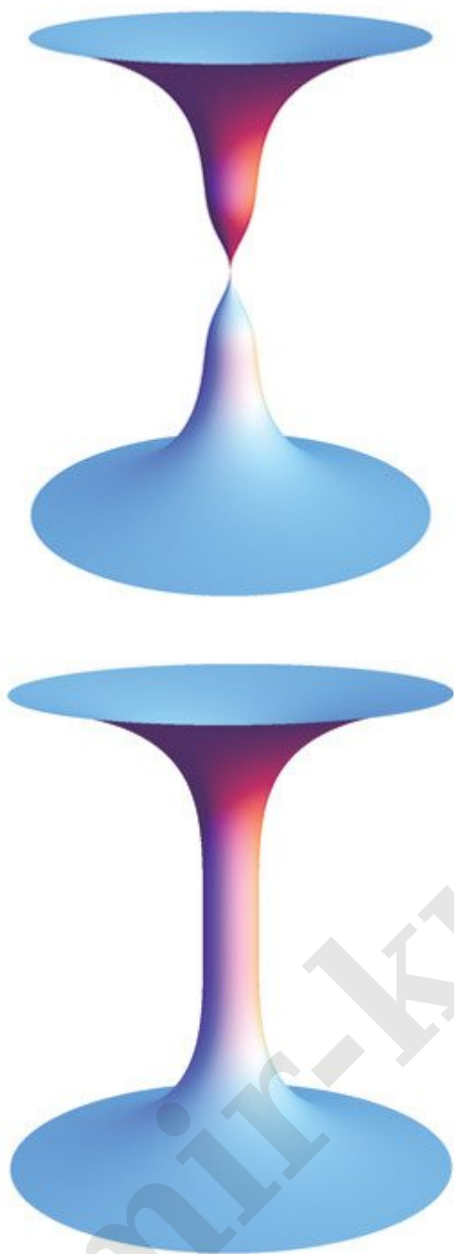
Рис. 25.5. Червоточины. Сверху: схлопывающаяся. Снизу: удерживаемая в открытом состоянии полями балка
