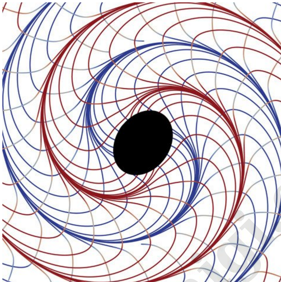
Рис. 16.7. Тендекс-линии вращающейся деформированной черной дыры (Рисунок Роба Оуэна.)
