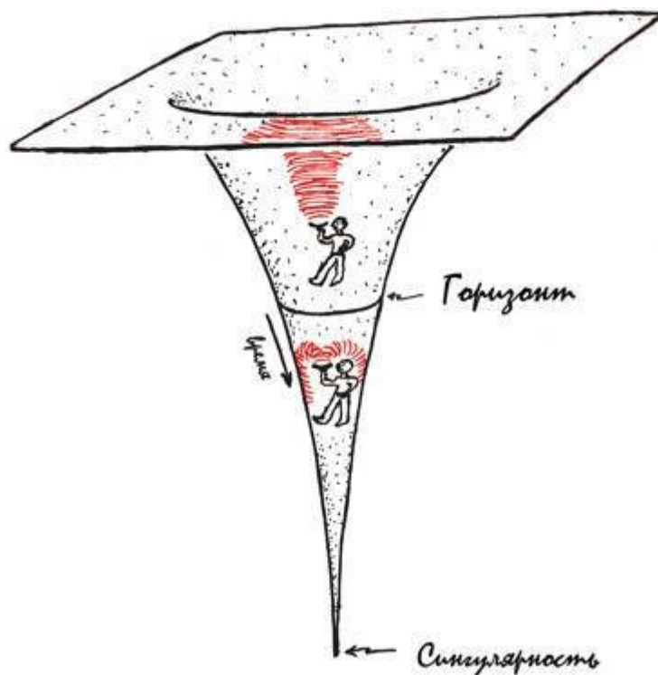
Рис. 5.3. Сигналы, которые я посылаю после пересечения горизонта событий, не могут выйти наружу. Важная оговорка: поскольку одно измерение тут опущено, я — двумерный Кип, скользящий по искривленной двумерной поверхности, части нашей браны (Мой набросок от руки.)
