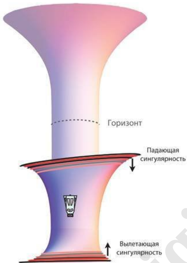
Рис. 28.2. «Рейнджер» зажат между падающей и вылетающей сингулярностями Гаргантюа. «Рейнджер» здесь гораздо больше, чем был бы в действительности
