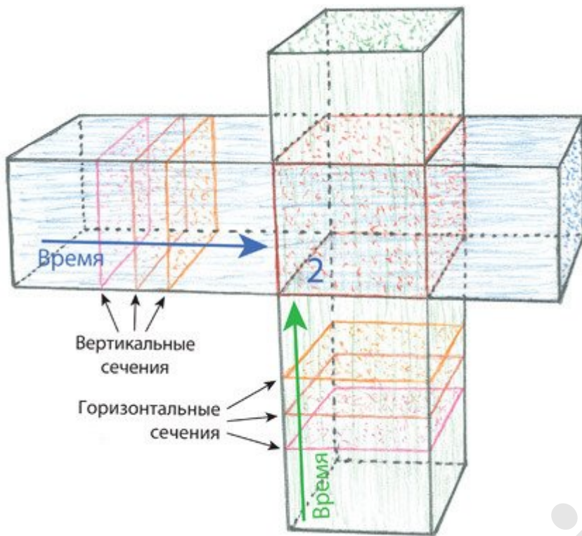
Рис. 29.12. Сечения спальни Мёрф движутся по двум стержням. Спальня 2 находится там, где пересекаются два набора сечений
