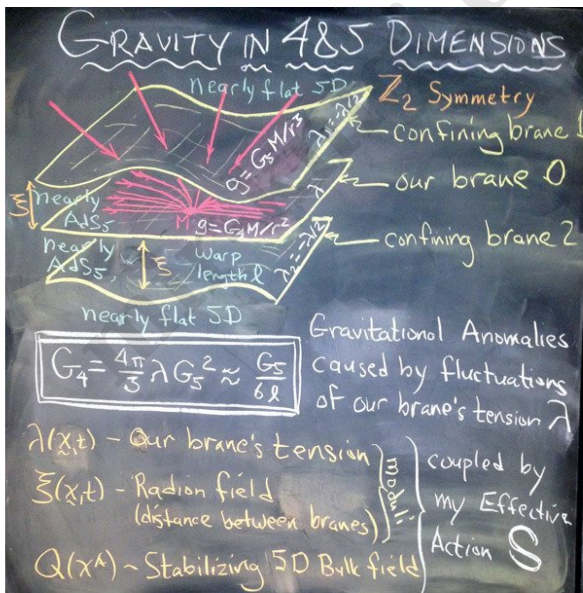
Рис. 3.6. Релятивистские уравнения на доске профессора Брэнда, описывающие возможные
