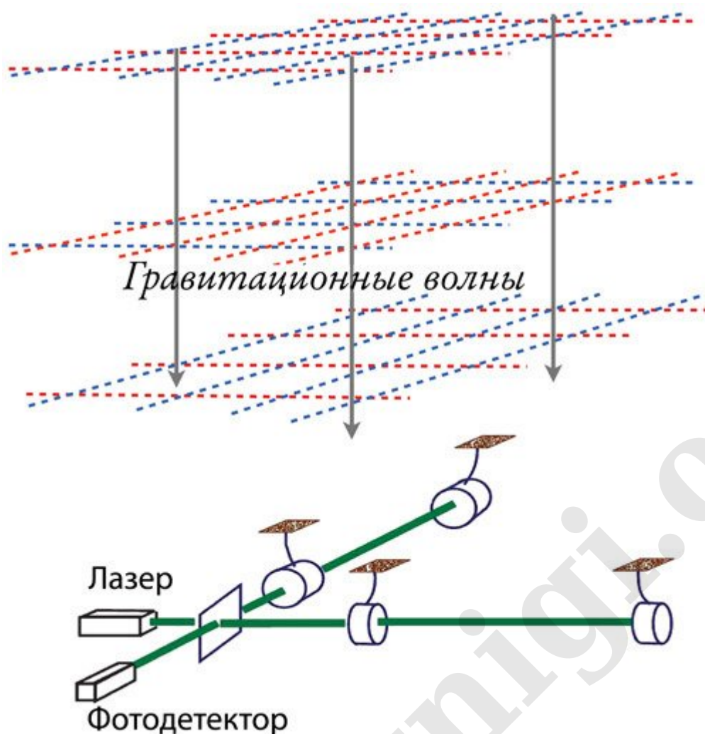
Рис. 16.8. Гравитационные волны, проходящие через детектор ЛИГО
