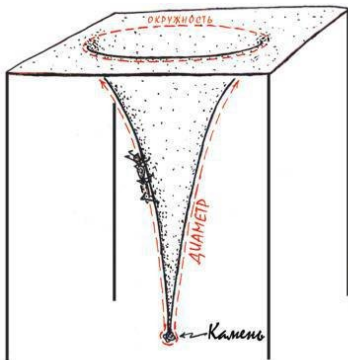
Рис. 5.1. Муравей на прогибающемся батуте (Мой набросок от руки.)
