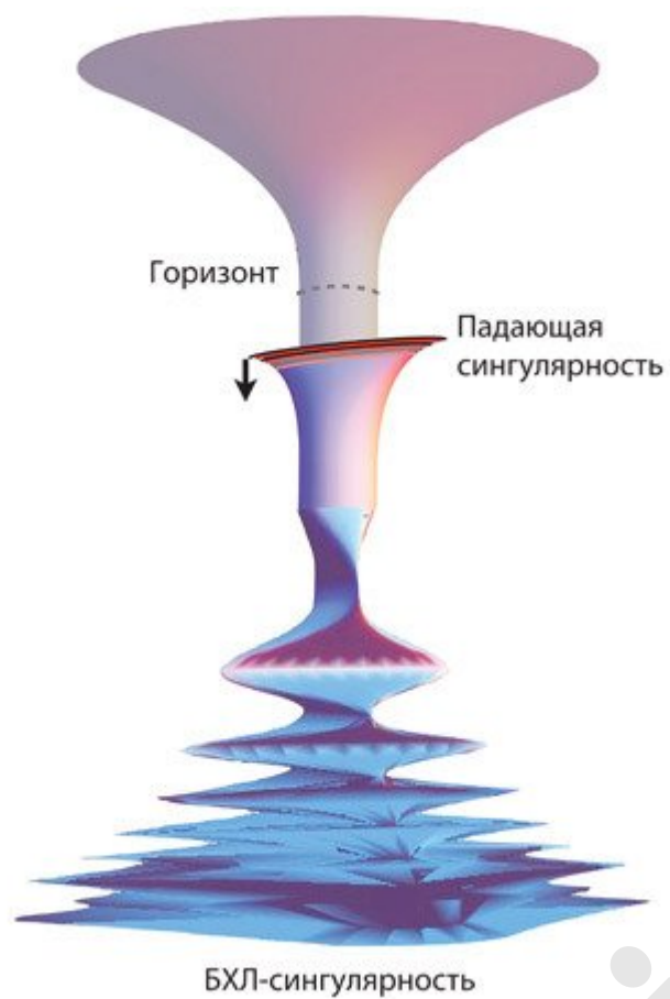
Рис. 26.11. Падающая сингулярность, порожденная всем тем, что падает в черную дыру (разноцветные ободки) вслед за вами
