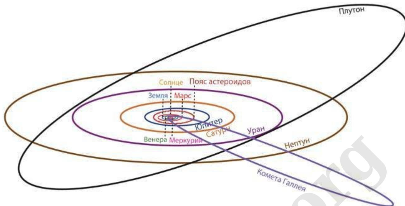
Рис. 7.5. Орбиты планет, Плутона и кометы Галлея в Солнечной системе — эллиптические
