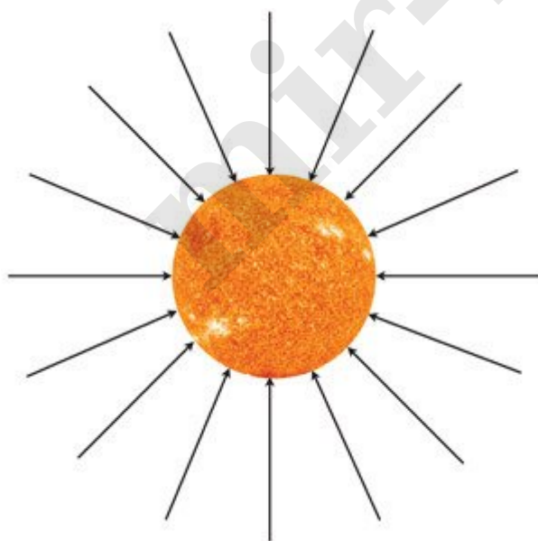
Рис. 23.1. Силовые линии гравитационного поля вокруг Солнца
