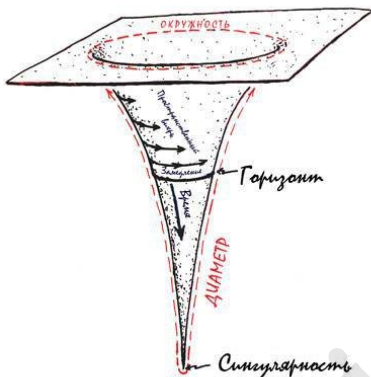
Рис. 5.4. Пространство вблизи вращающейся черной дыры затягивается в вихревую воронку (Мой набросок от руки.)
