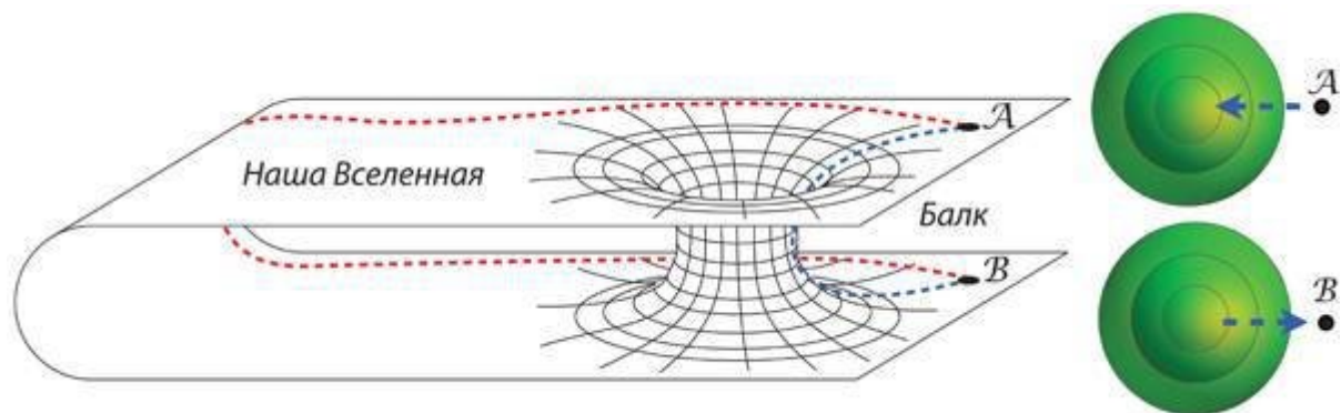
Рис. 14.2. Червоточина Фламма
