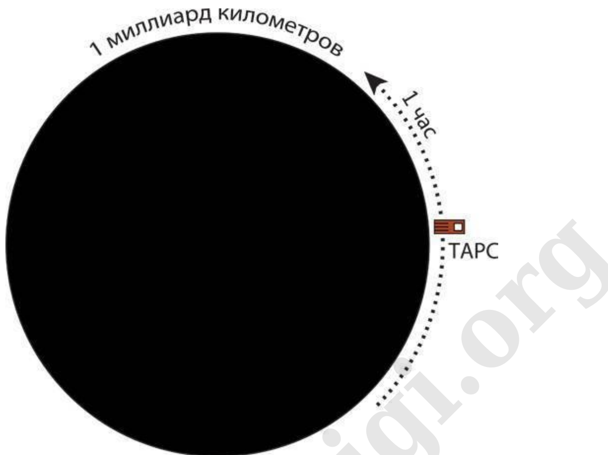
Рис. 6.2. TAPC, падающий к Гаргантюа, будет вращаться по окружности в миллиард километров; один оборот за час (для стороннего наблюдателя)
