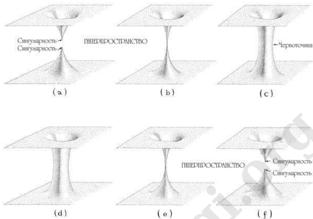
Рис. 14.3. Динамика червотчины Фламма (моста Эйнштейна — Розена) (Рисунок Мэтта Зимета по моему наброску; из книги [Торн 2009].)
