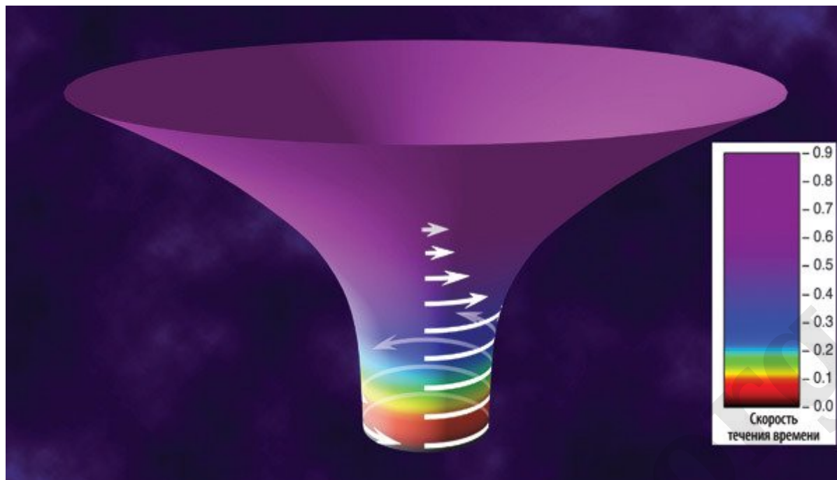
Рис. 5.5. Численно точное изображение искривления пространства и времени вблизи быстровращающейся черной дыры. Скорость вращения составляет 99,8 процента от максимально возможной (Рисунок Дона Дэвиса по моему наброску.)
