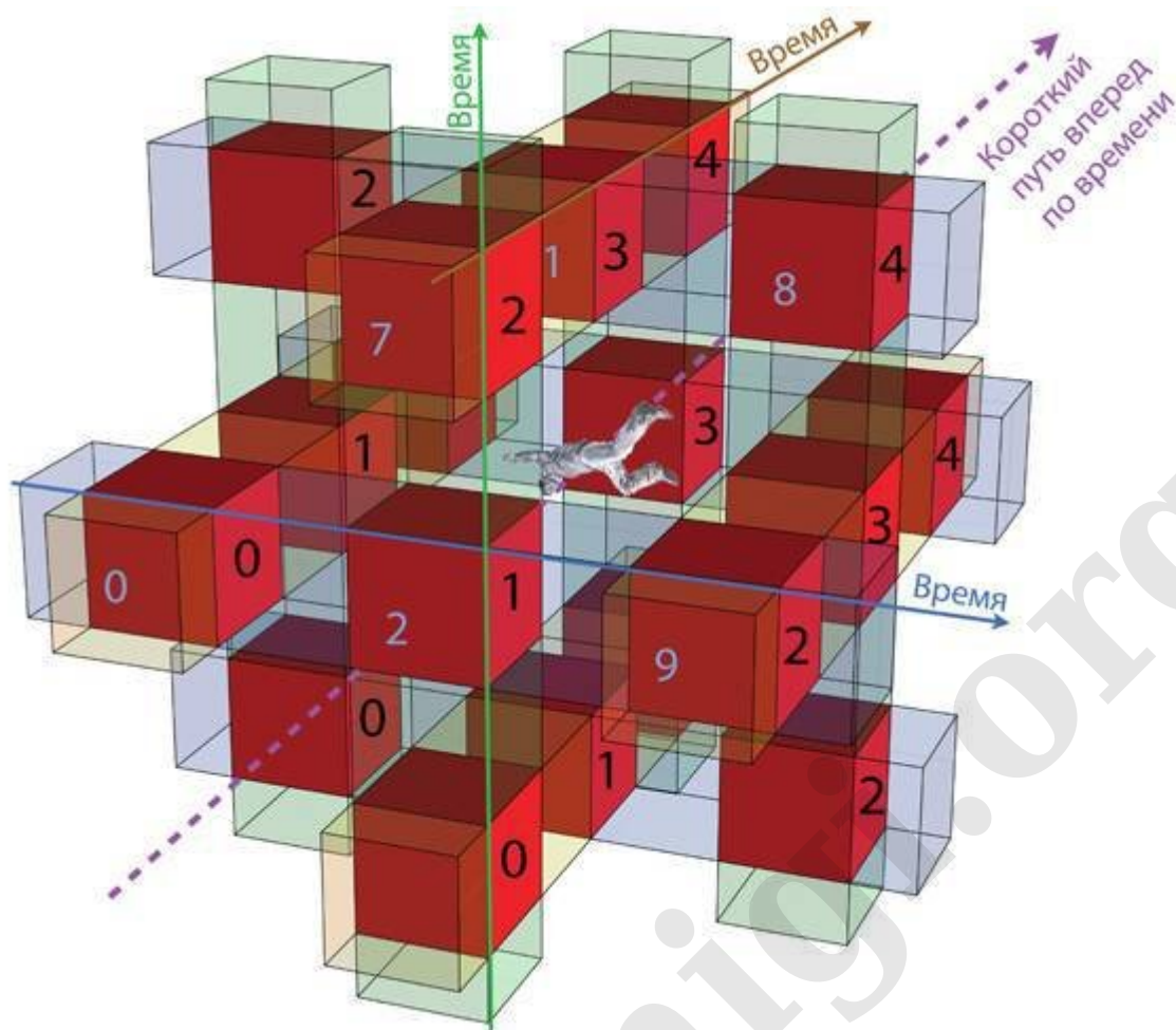
Рис. 29.13. Фрагмент решетки, образованной пересечениями движущихся по стержням сечений спальни. Голубыми числами обозначены спальни (сохраняется нумерация с предыдущих рисунков). Черные числа показывают количество секунд, на которое отстоит та или иная спальня от спальни 0. Пунктирная фиолетовая стрелка — направление, в котором Купер может быстрее всего продвинуться вперед по времени спальни
