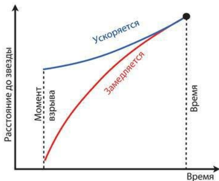
Рис. 24.4. Расстояние до звезды в момент взрыва (когда был испущен видимый нами свет) в двух вариантах: расширение Вселенной замедляется (красная кривая) или ускоряется (синяя). Наблюдаемый взрыв оказался тусклее, чем ожидалось, а значит дальше. Следовательно, Вселенная должна ускоряться
