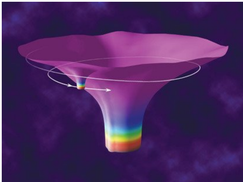
Рис. 21.1. Маленькая черная дыра, падающая по спирали в большую черную дыру: вид из балка, одно пространственное измерение опущено (Рисунок Дона Дэвиса по моему наброску.)
