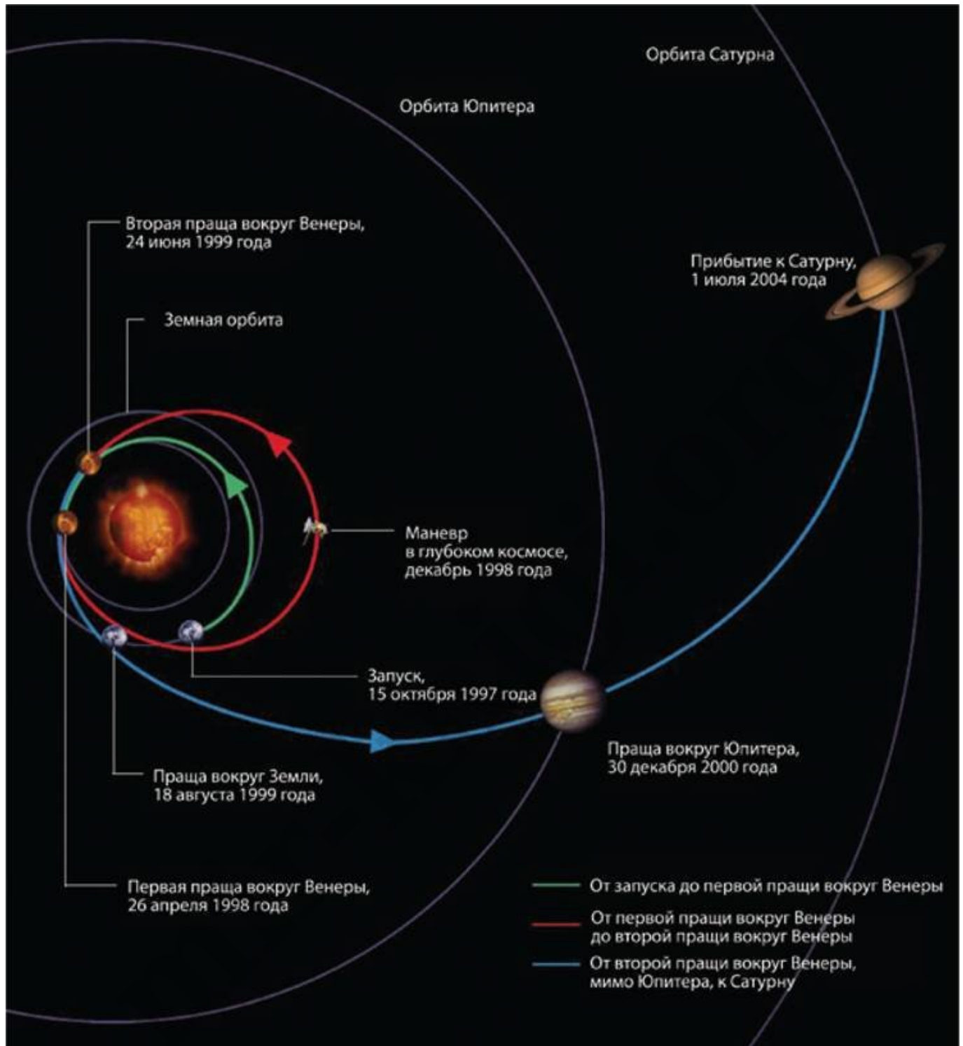
Рис. 7.7. Траектория полета «Кассини» от Земли до Сатурна
