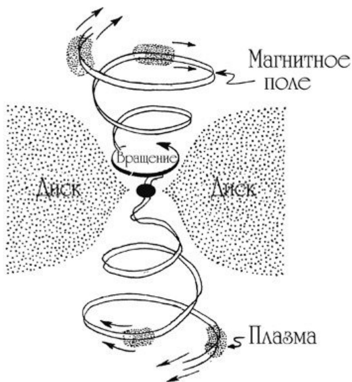
Рис. 9.3. Механизм образования джетов Блэндфорда — Знаека (Рисунок Мэтта Зимета по моему наброску; из [Торн 2009].)
