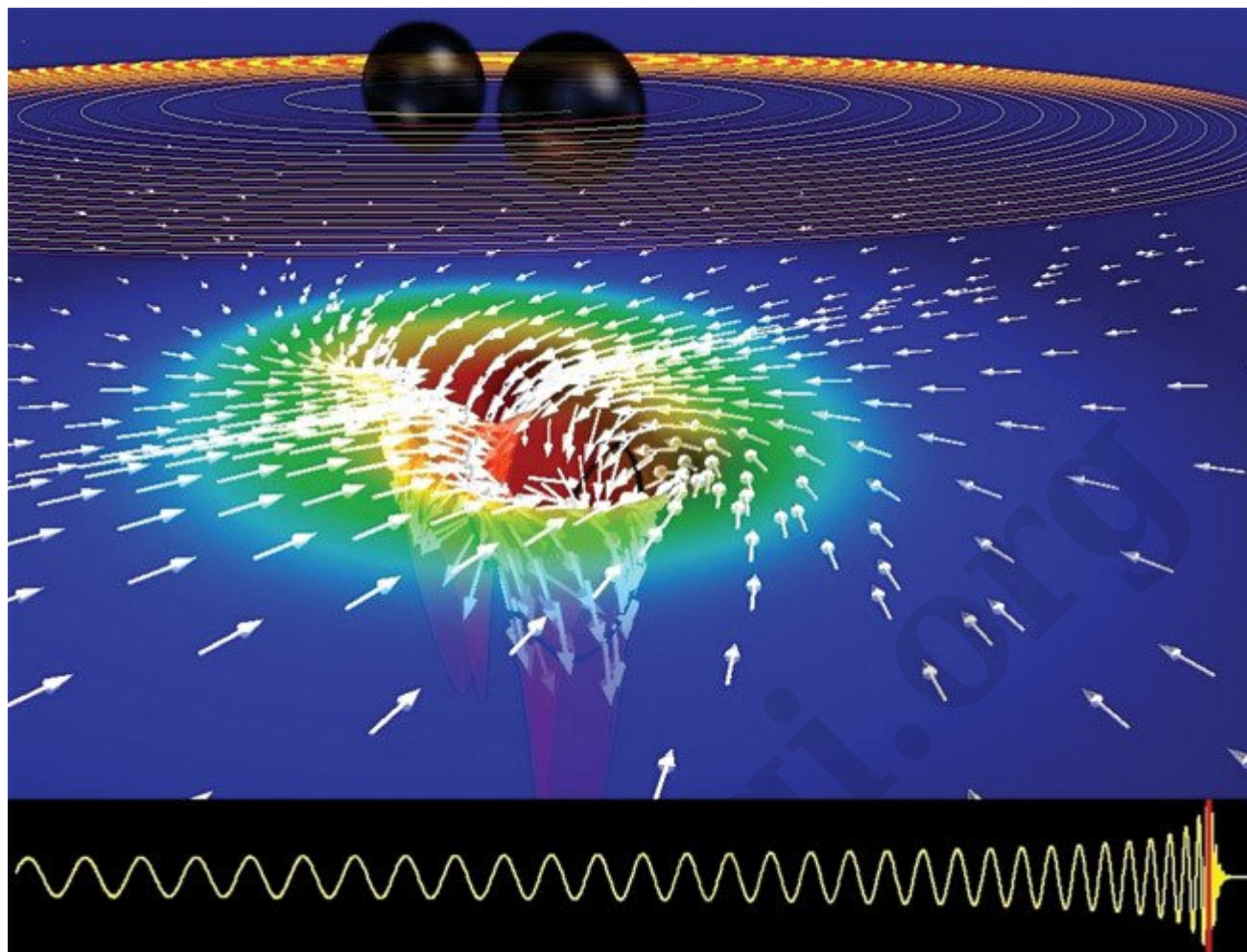
Рис. 16.9. Момент столкновения двух черных дыр. Модель для одинаковых невращающихся черных дыр. Сверху: орбиты и тени дыр, вид из нашей Вселенной. Посередине: искривленное пространство и время, вид из балка; стрелками показано, как пространство вовлекается в движение, а изменяющимися цветами — как искривляется время. Снизу: форма испускаемых гравитационных волн (Из фильма Гаральда Пфайфера о работе команды SXS.)
