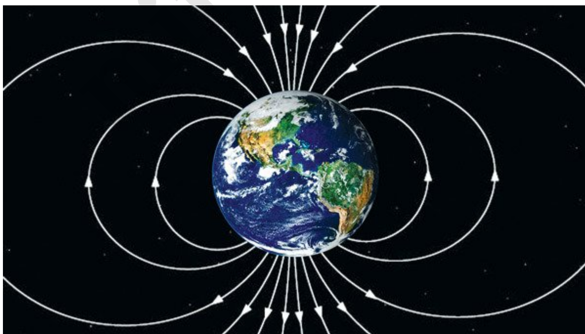
Рис. 2.8. Силовые линии магнитного поля Земли
