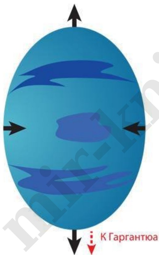
Рис. 17.3. Приливная деформация планеты Миллер
