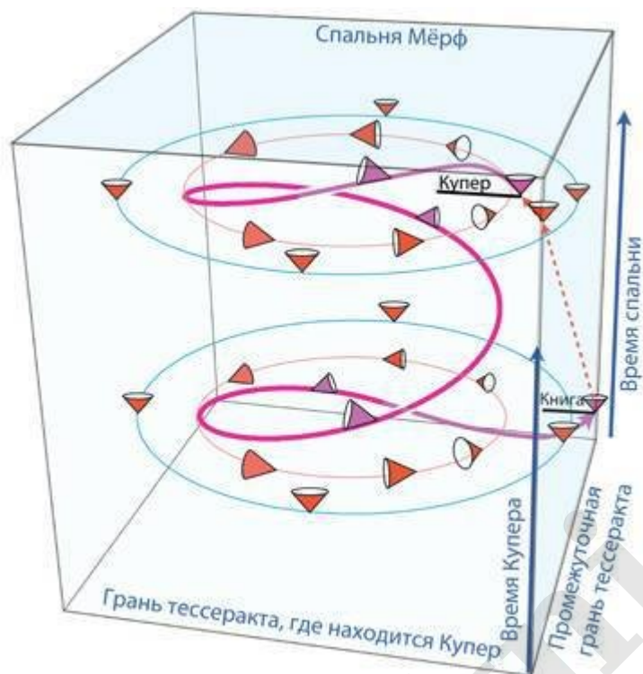
Рис. НТП. 1. Каузальная структура пространства — времени внутри тессеракта; одно пространственное измерение опущено
