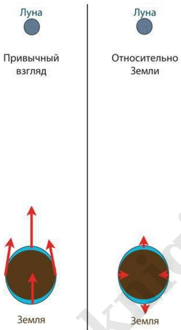
Рис. 4.8. Ньютоновское объяснение океанских приливов на Земле
