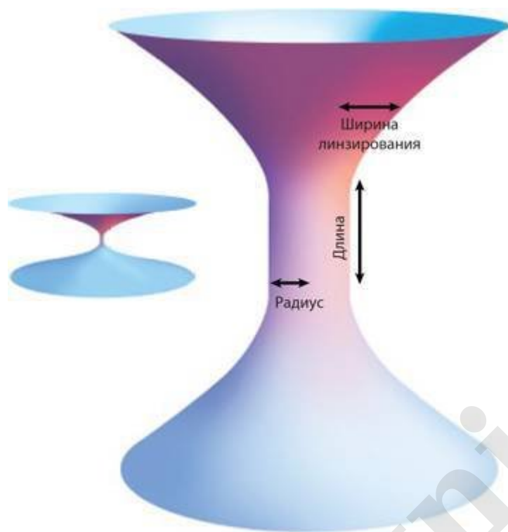
Рис. 15.1. Червоточина при взгляде из балка и три «ручки настройки» (Слева — та же червоточина в балке, но на большем отдалении, благодаря чему видна ее «расширенная версия».)
