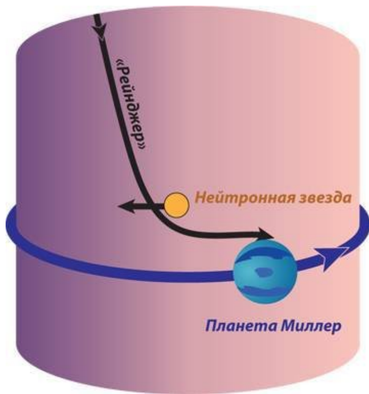
Рис. 7.3. Гравитационная праща вокруг нейтронной звезды позволяет совершить посадку на планету
