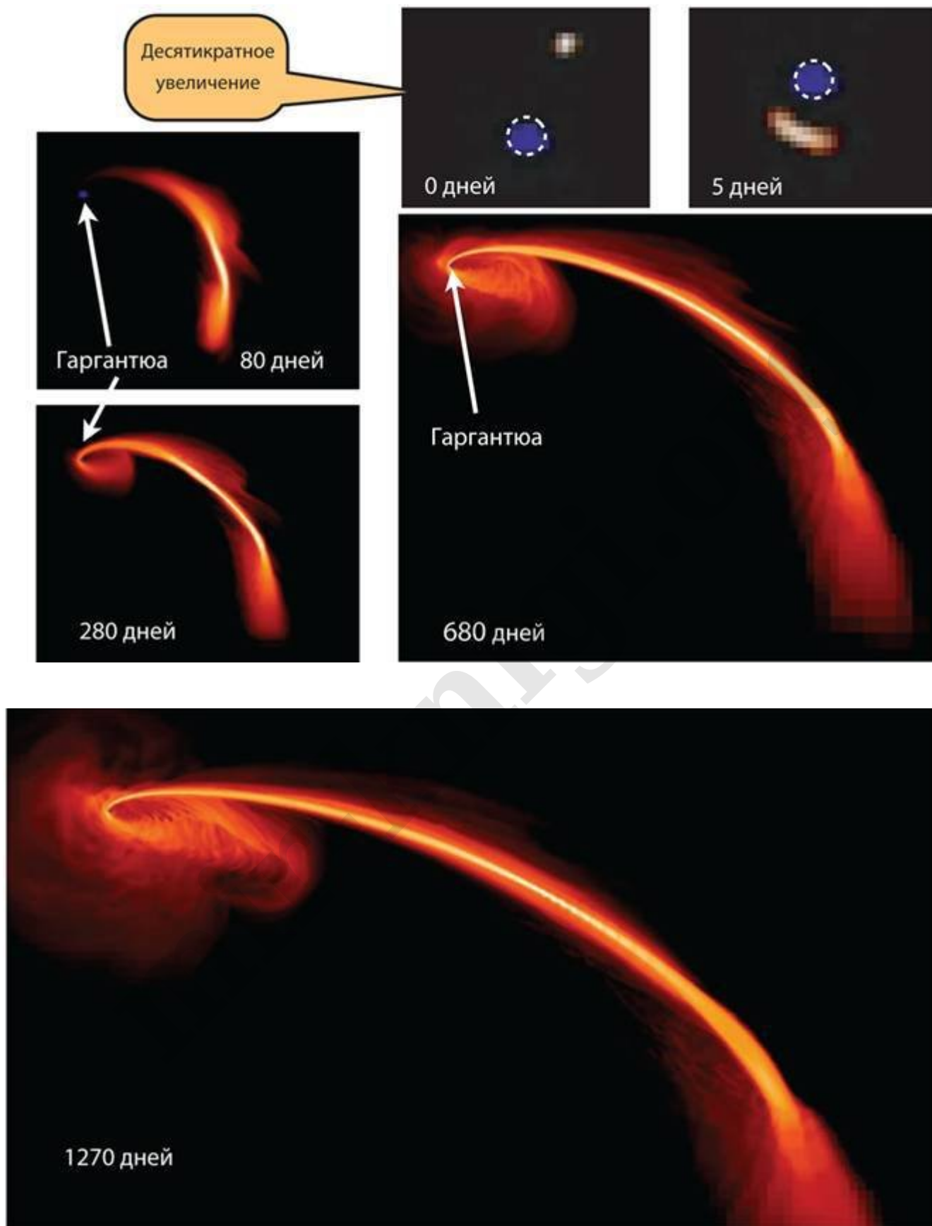
Рис. 9.6. Приливное разрушение звезды (красного гиганта) черной дырой Гаргантюа
