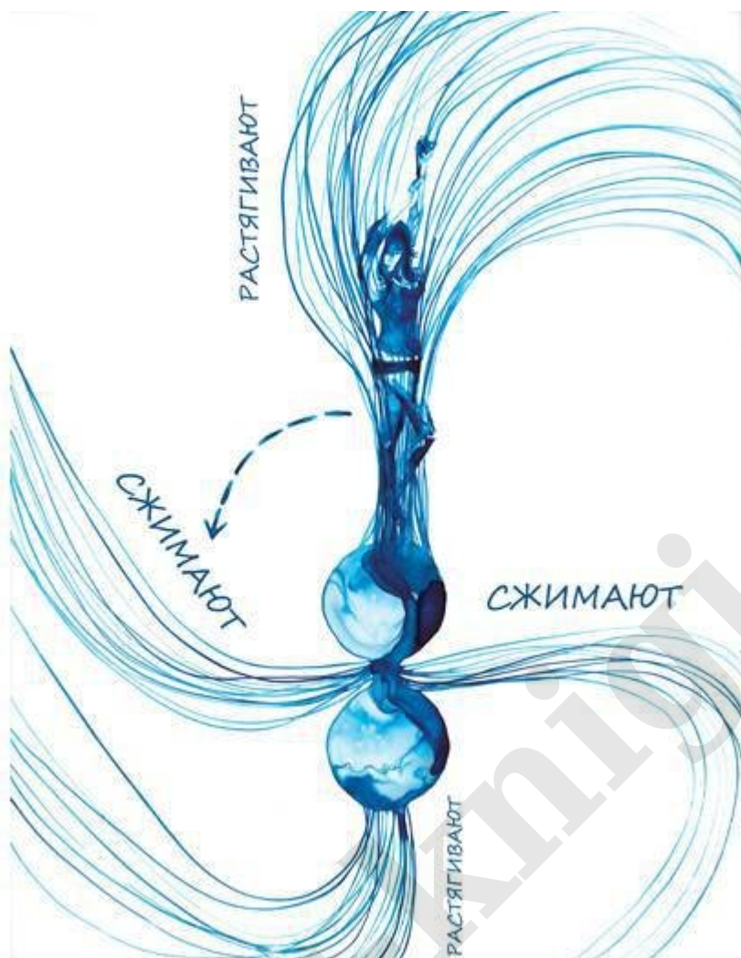
Рис. 16.6. Пара черных дыр, которые сталкиваются, вращаясь одна вокруг другой против часовой стрелки, и их тендекс-линии (Рисунок Лии Хэллоран.)
