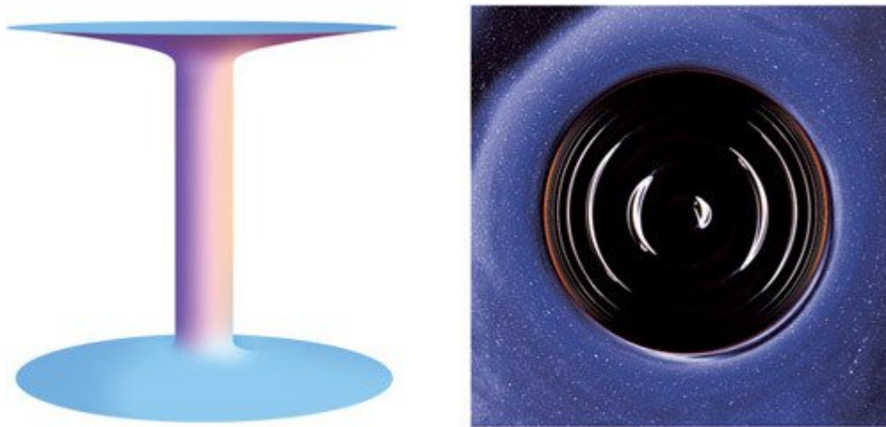
Рис. 15.2. Слева: три варианта червоточины с маленькой шириной линзирования (всего пять процентов от радиуса червоточины), вид из балка. Справа: то, что видит камера. Сверху вниз длина червоточины увеличивается: 0,01, 1 и 10 радиусов червоточины (Модели выполнены командой Эжени фон Танзелманн с помощью программы Оливера Джеймса, основанной на моих уравнениях.)
