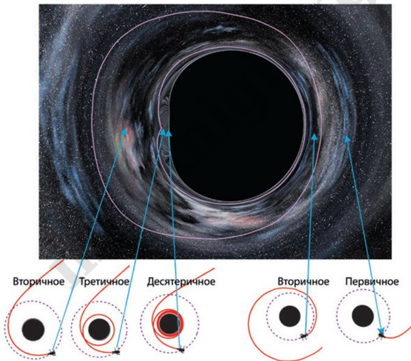
Рис. 8.6. Лучи света, формирующие изображения звезд, на которые указывают синие стрелки (Модель Double Negative, та же, что на рис. 8.1 и 8.5.)
