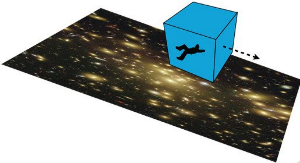
Рис. 29.4. Купер путешествует через балку, над нашей браной, в одной из граней тессеракта. Одно пространственное измерение опущено
