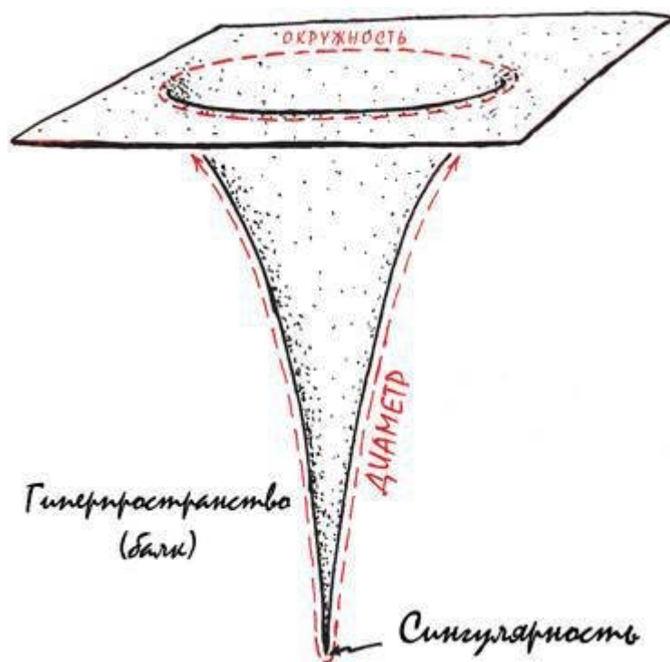
Рис. 5.2. Искривленное пространство внутри и вблизи черной дыры, взгляд из балка (Мой набросок от руки.)
