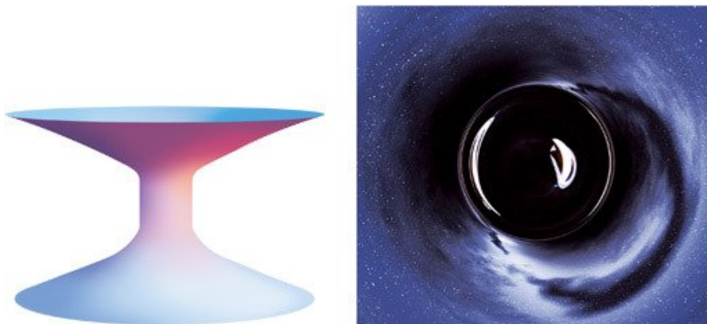
Рис. 15.4. Гравитационное линзирование звездного поля и Сатурна червоточиной для двух значений ширины линзирования: 0,014 (сверху) и 0,43 (снизу) радиуса червоточины (Модели выполнены командой Эжени фон Танзелманн с помощью программы Оливера Джеймса, основанной на моих уравнениях.)
