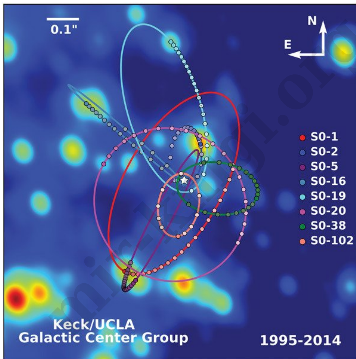
Рис. 5.8. Наблюдаемые орбиты движения звезд вокруг массивной черной дыры, находящейся в центре галактики Млечный Путь. Данные наблюдений Андреа Гез и ее коллег
