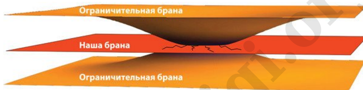
Рис. 25.6. Столкновение бран
