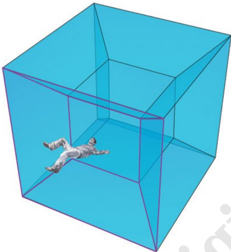
Рис. 29.3. Купер внутри трехмерной грани тессеракта
