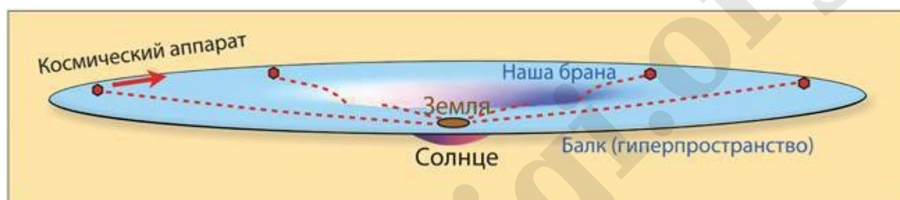
Рис. 4.4. Траектории пути радиосигналов от аппаратов «Викинг» через искривленную экваториальную плоскость Солнца
