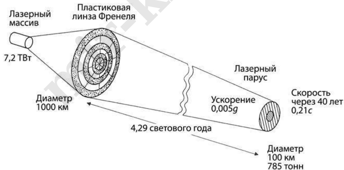
Рис. 13.3. Механизм передвижения с помощью лазерного луча и светового паруса Роберта Форварда [Forward 1984]
