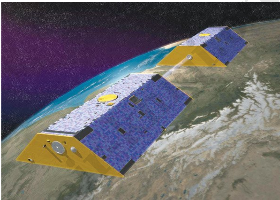
Рис. 24.8. GRACE: два спутника, каждый из которых отслеживает положение другого с помощью микроволновых сигналов, сближаются и отдаляются под действием тендекс-линий (на рисунке не показаны)
