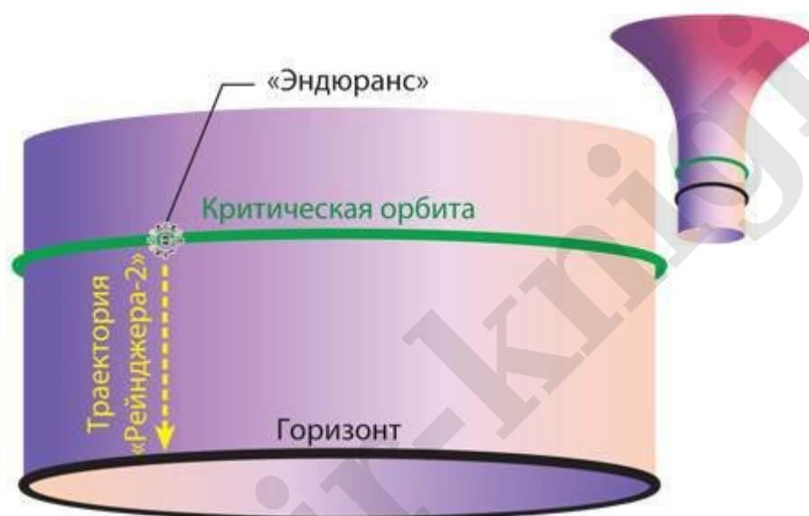
Рис. 28.1. Траектория, по которой «Рейнджер» движется через искривленное пространство Гаргантюа, в орбитальной системе отсчета «Эндюранс» (корабль изображен большим, чем он есть в действительности, чтобы вы могли его разглядеть). В правом верхнем углу: более крупная область искривленного пространства Гаргантюа (Изображение «Эндюранс» взято из фильма.)
