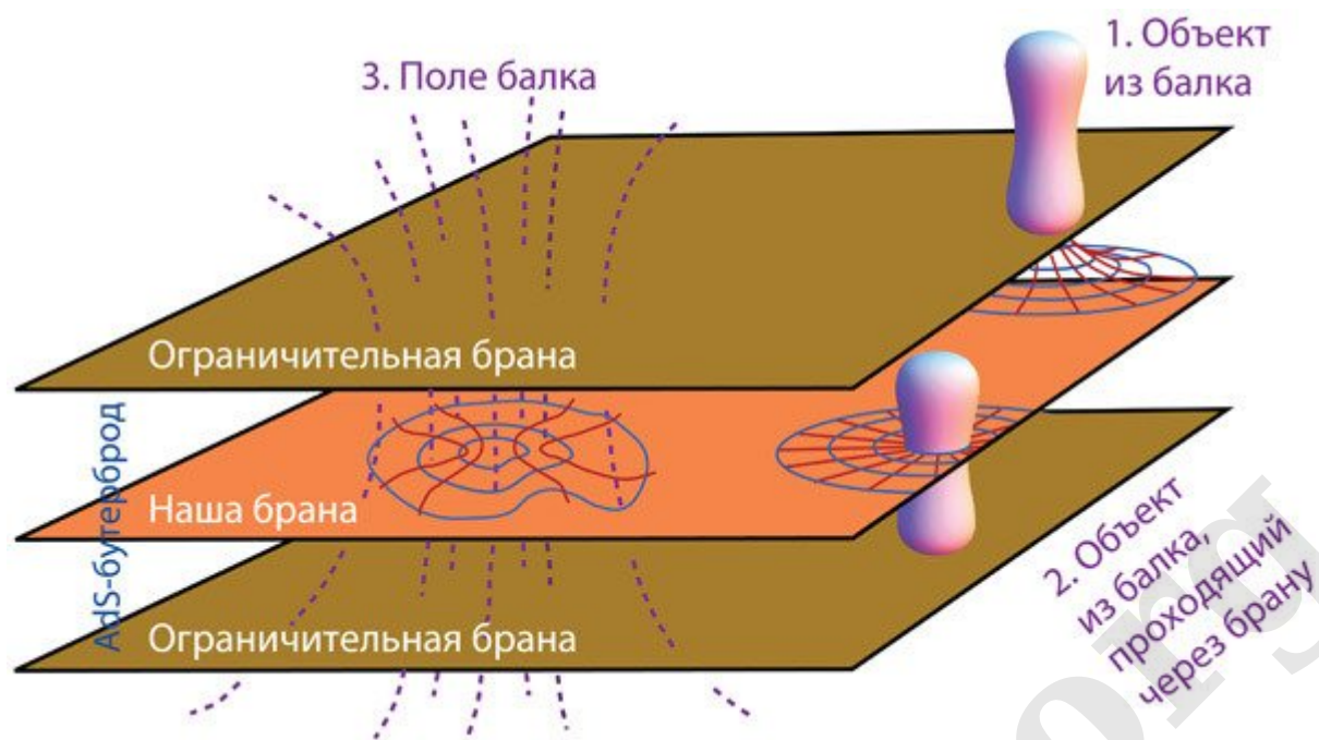
Рис. 25.3. Три способа, которыми балк может вызвать наблюдаемые гравитационные аномалии. Красные и синие кривые — приливные тендекс-линии, порождаемые объектом из балка или полем балка
