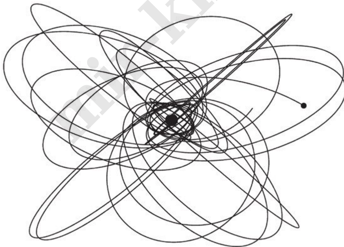
Рис. 10.1. Типичная орбита объекта, движущегося вокруг быстровращающейся черной дыры вроде Гаргантюа (Модель Стива Драско.)
