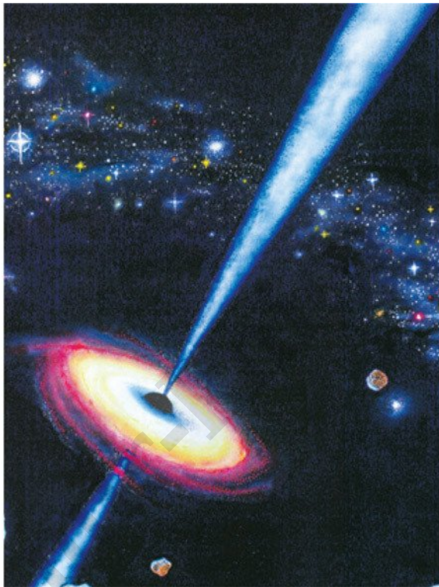
Рис. 9.2. Художественное изображение аккреционного диска черной дыры, а также джетов, образующихся около ее полюсов (Работа Мэтта Зимета по моему наброску; из [Торн 2009].)
