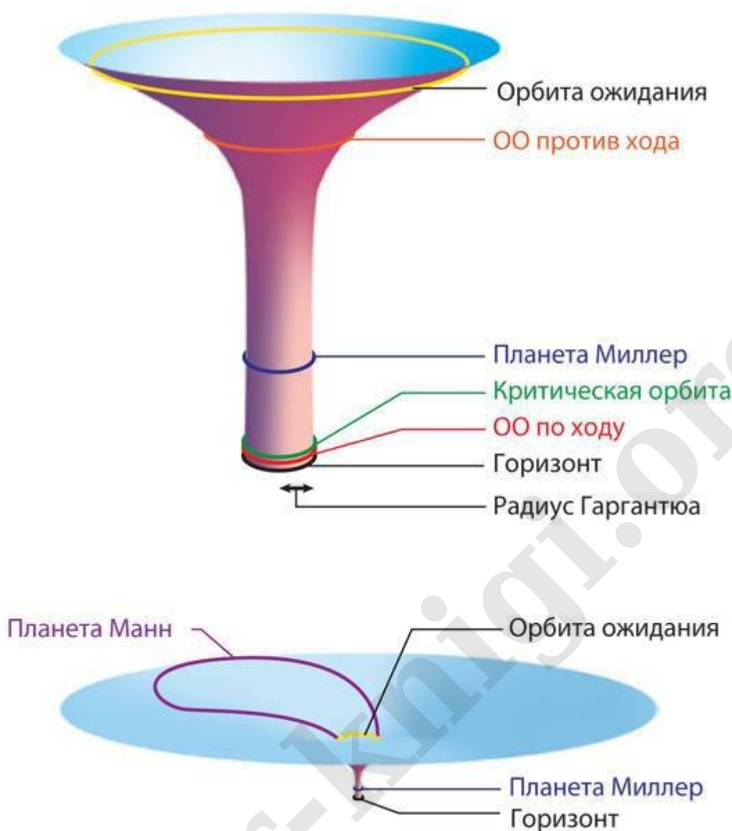
Рис. 6.3. Анатомия Гаргантюа при скорости вращения на одну стотриллионную меньше предельной (что необходимо для радикального замедления времени на планете Миллер)
