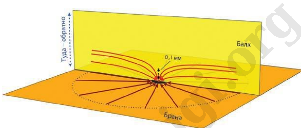
Рис. 23.6. Если в балке происходит AdS-искривление, силовые линии гравитационного поля изгибаются, выстраиваясь параллельно бране, поскольку пространство, в котором они могут распространяться над браной, ограничено (Перерисовка с иллюстрации из [Рэндалл 2011].)
