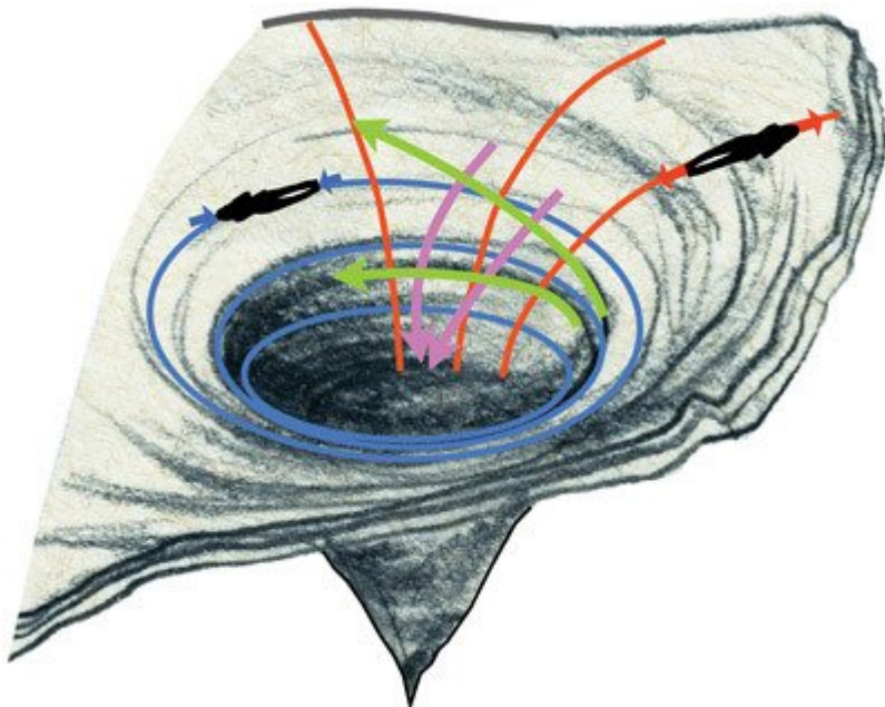
Рис. 4.7. Тендекс-линии вокруг черной дыры. Изображение дыры взято с рисунка Лии Хэллоран (рис. 4.5)
