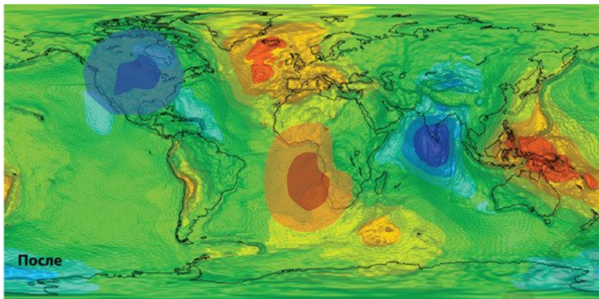
Рис. 25.4. Карты гравитационного притяжения Земли. Сверху: в 2014 году, по данным спутника GOCE. Снизу: после внезапного изменения в эпоху аномалий
