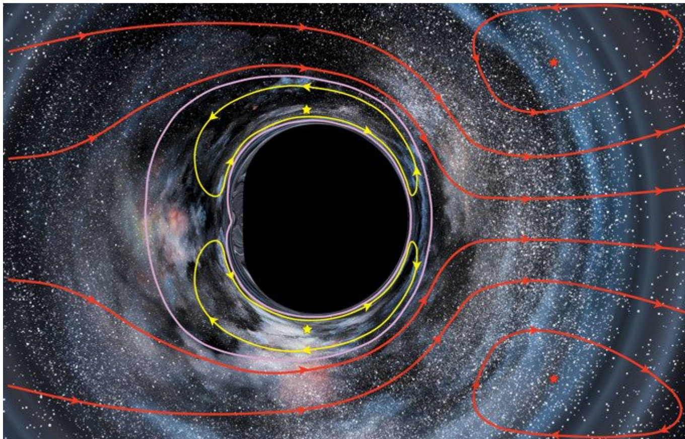
Рис. 8.5. Эффект перетекания звезд рядом с быстровращающейся черной дырой, подобной Гаргантюа, «вид через камеру». В этой модели студии Double Negative дыра вращается со скоростью в 99,9 процента от предельной, а камера движется по круговой экваториальной орбите, окружность которой в шесть раз превышает окружность горизонта. См. видеоролик на странице Interstellar.withgoogle.com
