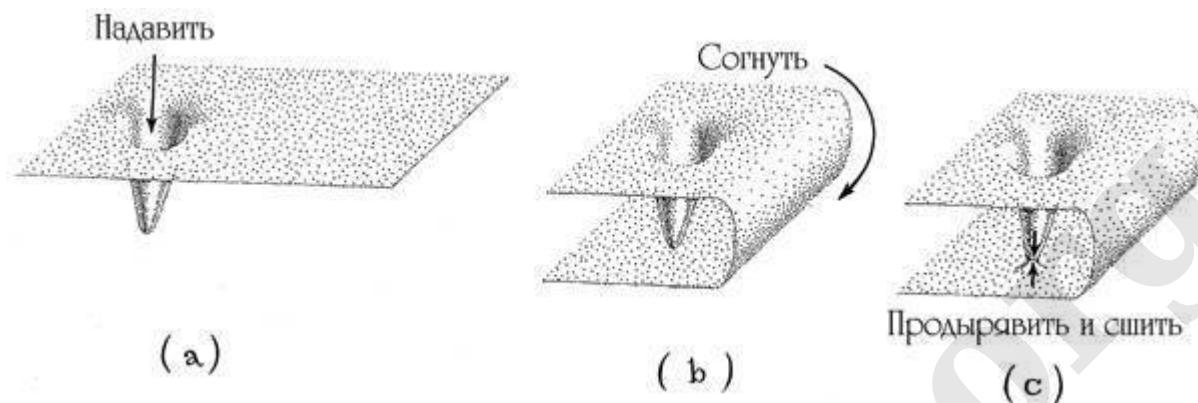
Рис. 14.8. Создание червоточины (Рисунок Мэтта Зимета по моему наброску; из [Торн 2009].)
