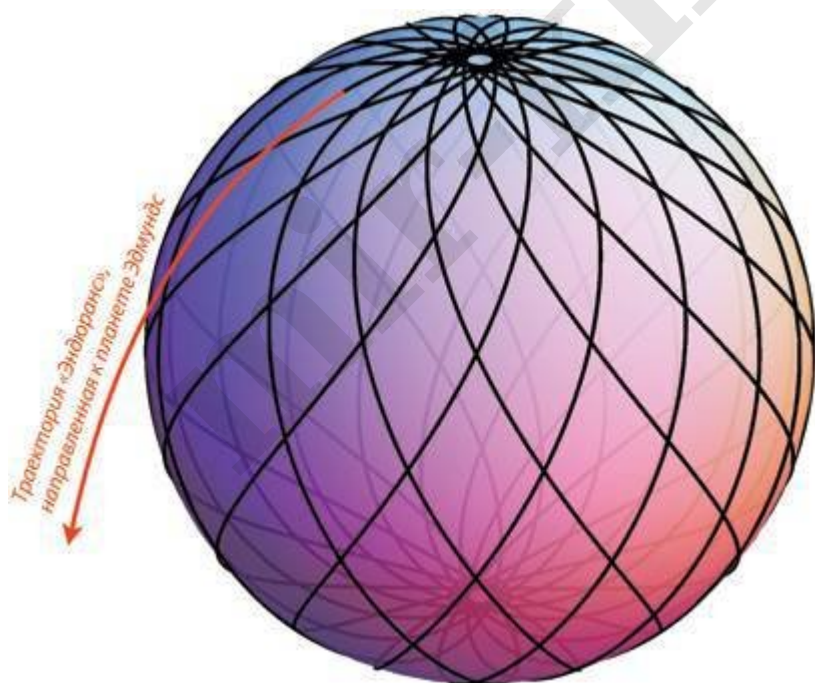
Рис. 27.10. Критическая орбита «Эндюранс» и запуск к планете Эдмундс в трех измерениях. Критическая орбита охватывает сферу, окружающую Гаргантюа
