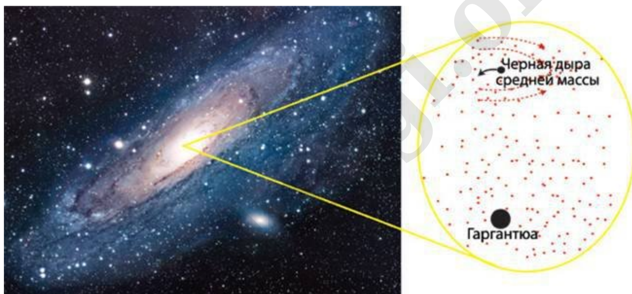
Рис. 7.4. Слева: галактика Андромеды, в ядре которой скрывается черная дыра размером с Гаргантюа. Справа: динамическое трение, благодаря которому дыра средней массы постепенно замедляется и притягивается все ближе к гигантской черной дыре
