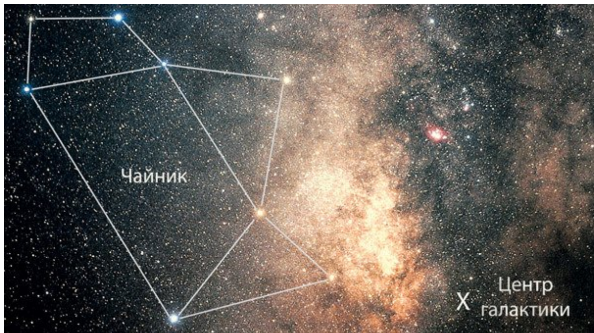
Рис. 5.9. Положение центра нашей галактики на ночном небе. Там находится гигантская черная дыра
