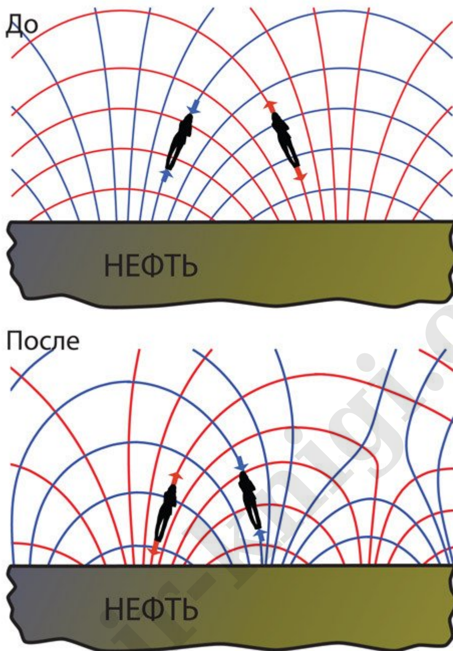
Рис. 25.2. Тендекс-линии (см. главу 4) приливной гравитации над нефтяным месторождением до и после внезапных изменений
