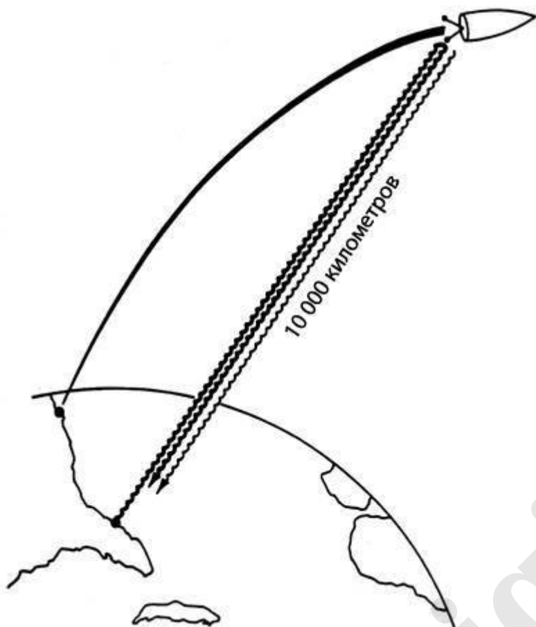
Рис. 4.1. Определение замедления времени на Земле с помощью атомных часов (из книги Клиффорда Уилла «Был ли прав Эйнштейн? Проверка общей теории относительности» [Will 1993])
