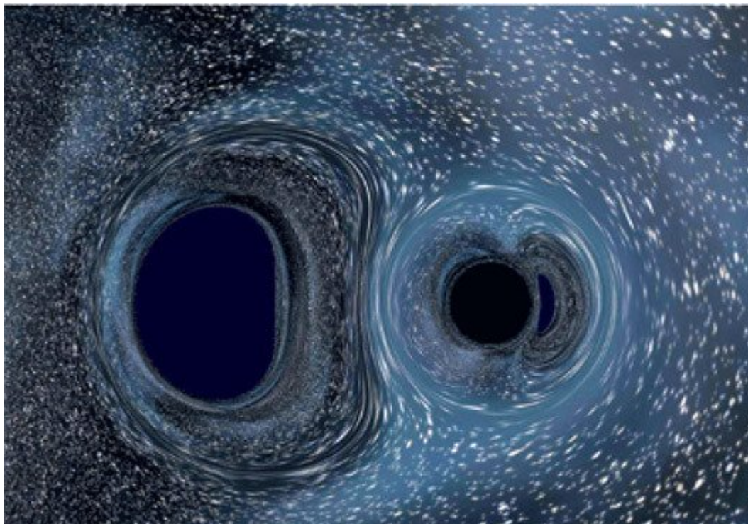
Рис. 8.7. Гравитационная праща вокруг дыры средней массы, на фоне Гаргантюа, вид с «Рейнджера» (Моя модель.)
