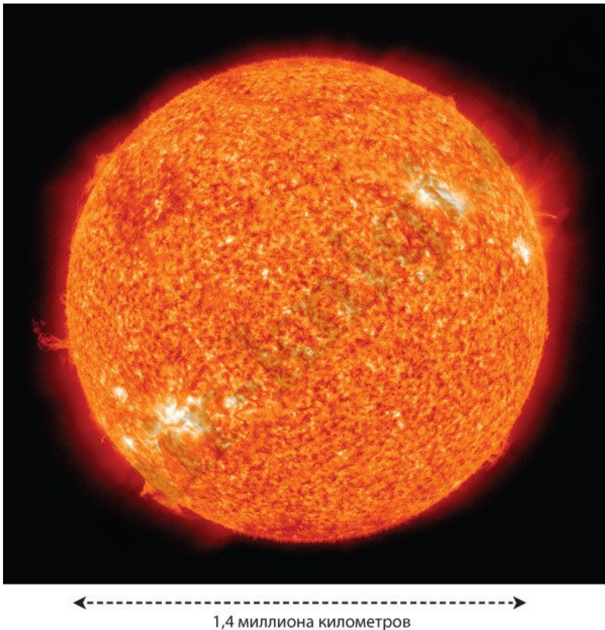
Рис. 2.3. Солнце, сфотографированное Обсерваторией солнечной динамики NASA
