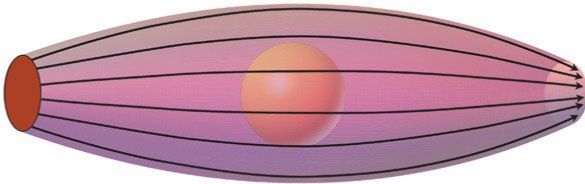
Рис. 14.5. Солнце (или черная дыра) сводит лучи света
