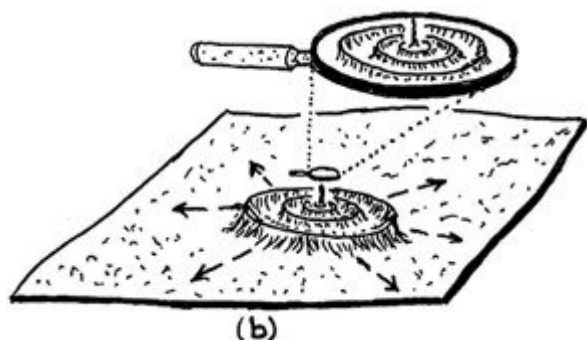
Рис. 26.7. Сверху: Мэттью Чоптюк. В центре (а): схлопывающаяся гравитационная волна. Снизу (b): кипение, вызванное волной, и голая сингулярность в центре увеличительного стекла
