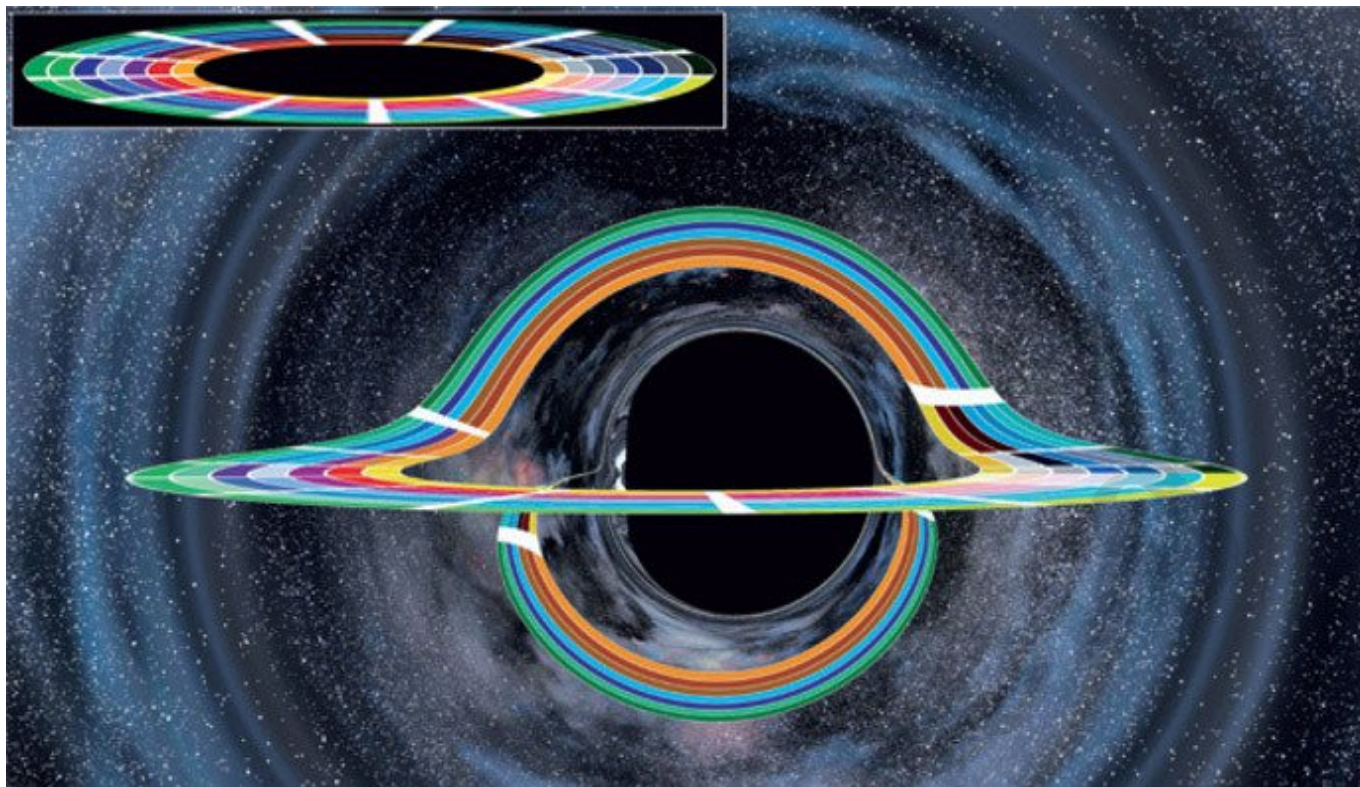
Рис. 9.7. Бесконечно тонкий диск в экваториальной плоскости Гаргантюа, гравитационно линзированный искривленным пространством и временем дыры. Гаргантюа здесь вращается очень быстро. Врезка: тот же диск без черной дыры (Изображение от команды Эжени фон Танзелманн из студии Double Negative.)
