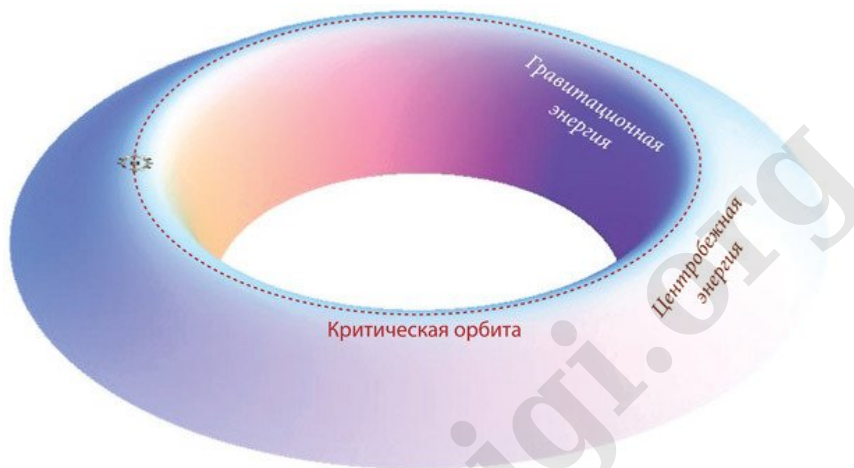
Рис. 27.5. Критическая орбита «Эндюранс» на кромке кратера. Центробежная энергия и центробежная сила преобладают снаружи от кратера, а отрицательная гравитационная энергия и сила гравитации — внутри него
