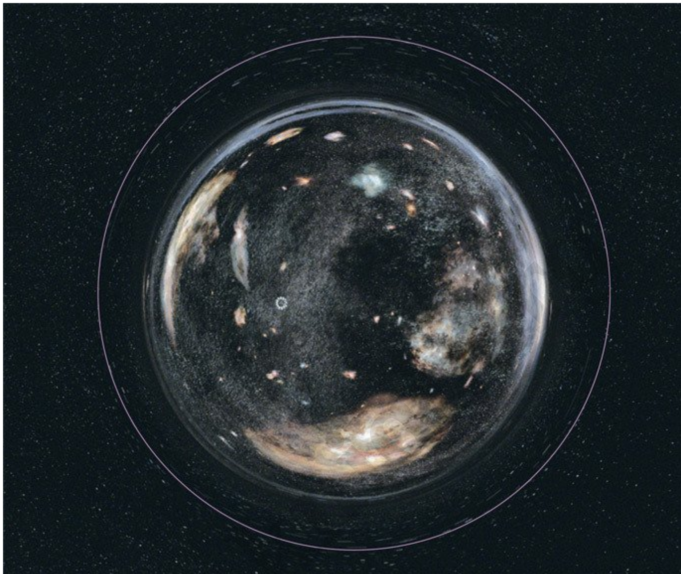
Рис. 15.5. Червоточина, как она показана в трейлере фильма. Перед червоточиной, ближе к центру, виден «Эндюранс». Фиолетовая окружность, которой я обвел червоточину, обозначает кольцо Эйнштейна, подобное кольцу на рис. 8.4 для невращающейся черной дыры. Первичные и вторичные изображения линзированных звезд здесь движутся таким же образом, как на рис. 8.4. Можете, посмотрев трейлер, проследить эти движения? (Кадр из «Интерстеллар», с разрешения «Уорнер Бразерс».)
