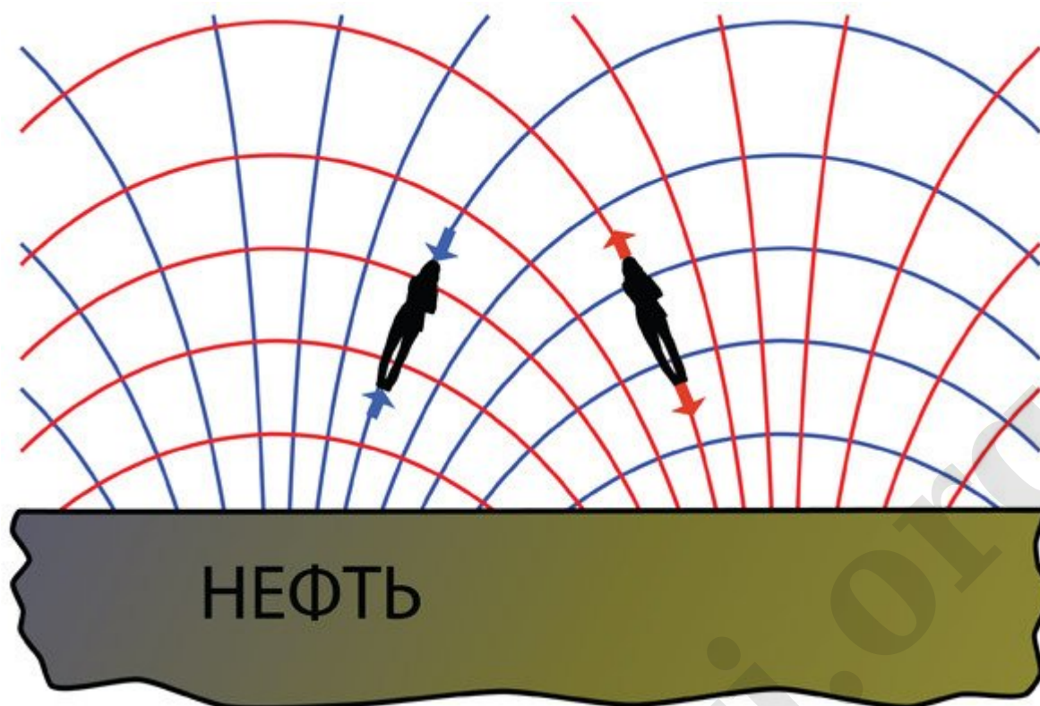
Рис. 24.6. Тендекс-линии над участком земной коры. Вдоль красных линий действует приливное растяжение, вдоль синих — сжатие
