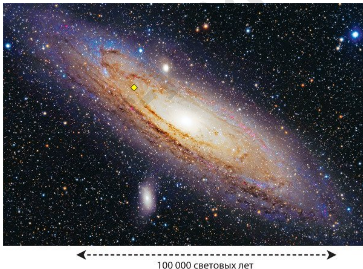
Рис. 2.2. Галактика Андромеды
