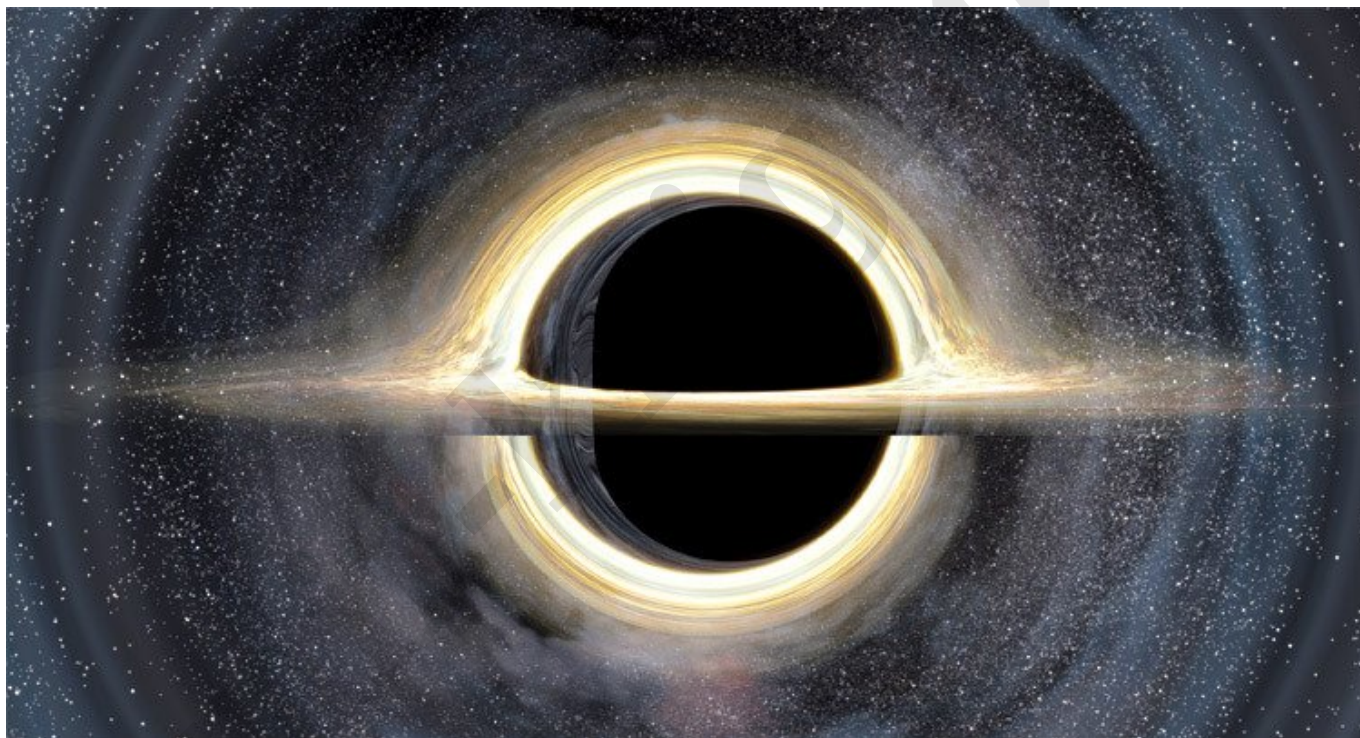
Рис. 9.9. Гаргантюа с более реалистичным бесконечно тонким аккреционным диском вместо цветного диска с рис. 9.7 (Изображение от команды Эжени фон Танзелманн из студии Double Negative.)
