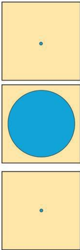
Рис. 22.2. Трехмерная сфера проходит через двумерную брану
