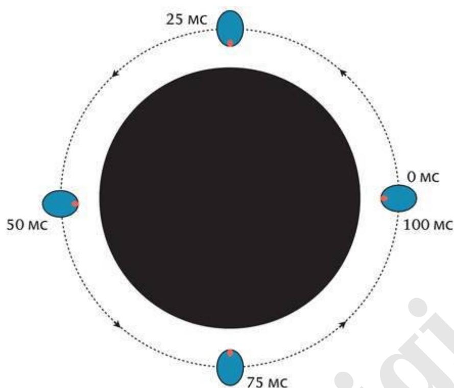
Рис. 17.4. Орбитальное движение и вращение планеты Миллер относительно отдаленных звезд. Красная точка на поверхности планеты и приливная выпуклость всегда направлены к Гаргантюа
