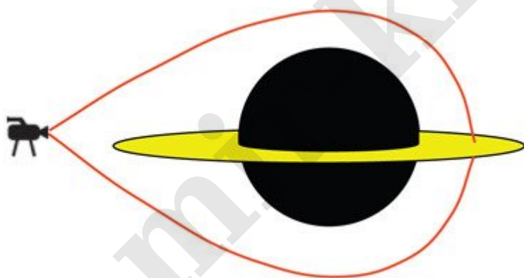
Рис. 9.8. Лучи света (красные линии), формирующие для камеры изображения области аккреционного диска, которая находится позади Гаргантюа: одно изображение — над тенью дыры, другое — под ней
