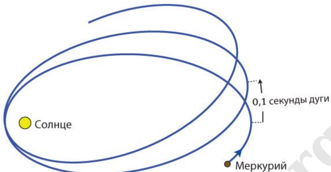
Рис. 24.1. Аномальная прецессия орбиты Меркурия. Я утрировал эллиптичность орбиты и величину прецессии
