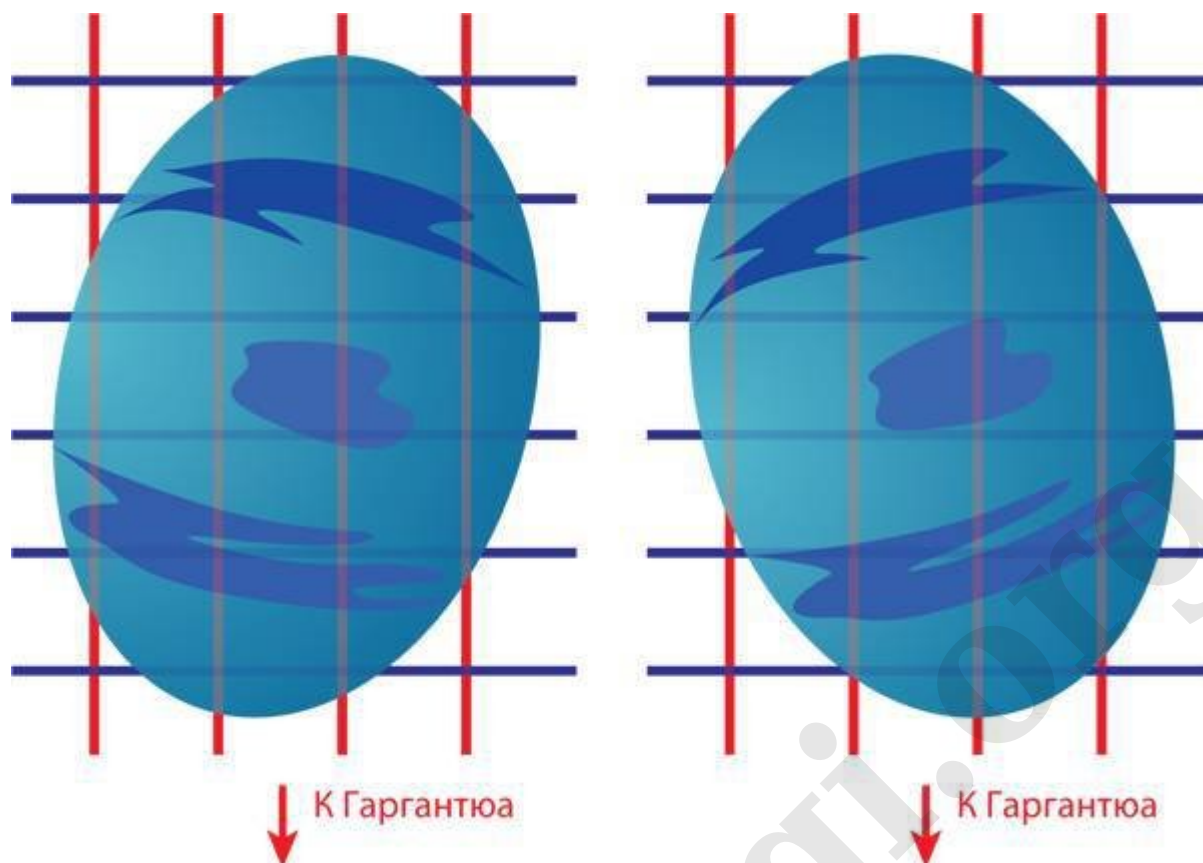
Рис. 17.6. Раскачивание планеты Миллер под воздействием приливной гравитации Гаргантюа, а именно ее растягивающих (красных) и сжимающих (синих) тендекс-линий
