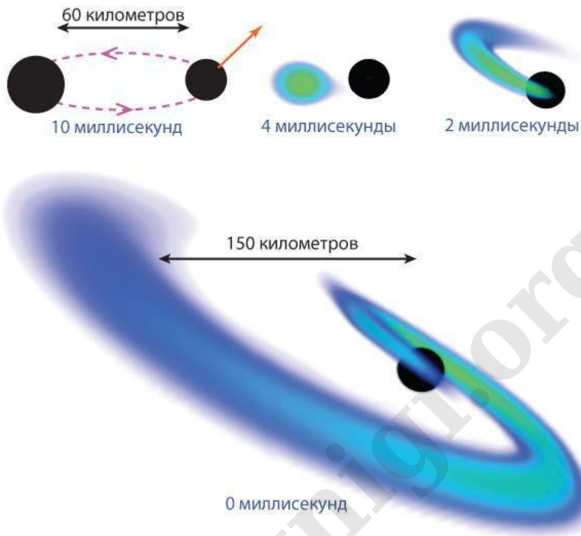
Рис. 16.4. Последние миллисекунды жизни нейтронной звезды (Модель Франсуа Фукара и коллег, см. black-holes.org .)
