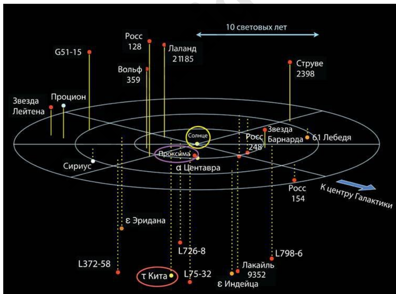
Рис. 13.1. Все звезды в пределах 12 световых лет от Земли. Солнце, проксима Центавра и тау Кита обведены кружками — желтым, фиолетовым и красным соответственно (Слегка
