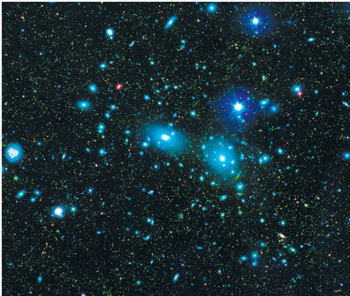
Рис. 24.2. Галактическое скопление Кома, увиденное через сильный телескоп
