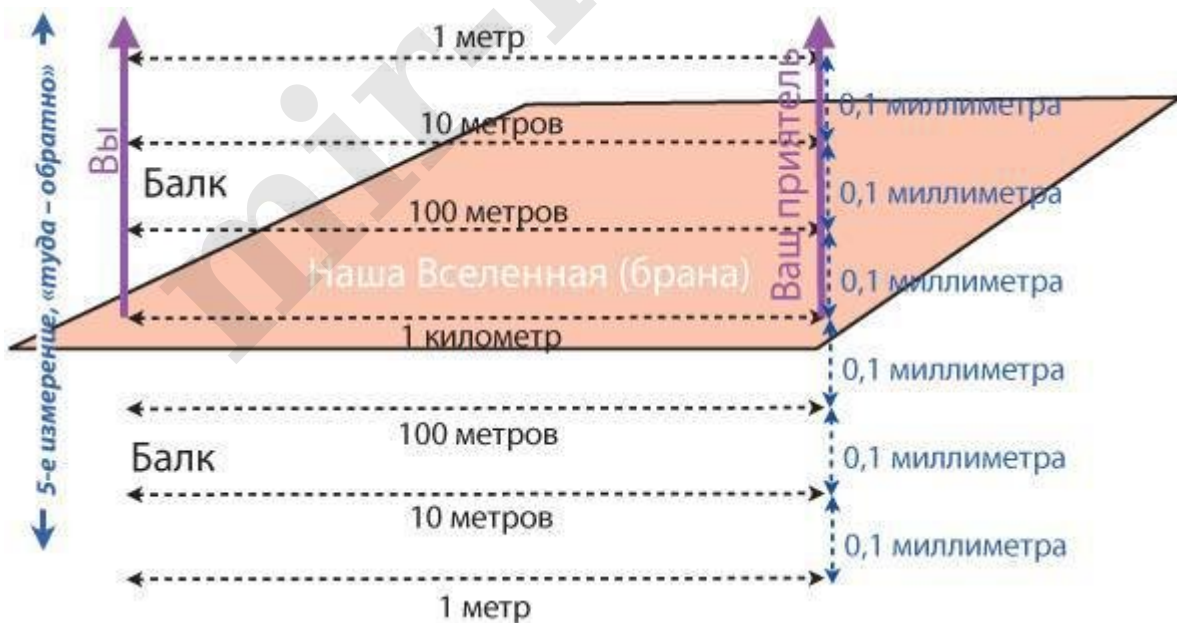
Рис. 23.5. AdS-искривление балка
