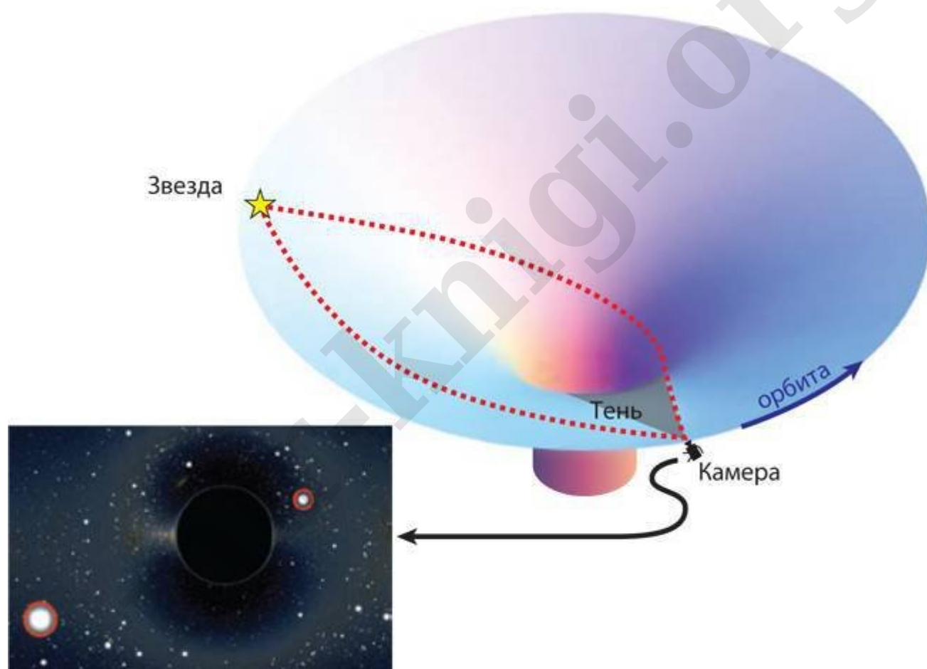
Рис. 8.3. Сверху: искривленное пространство вокруг невращающейся черной дыры (взгляд из балка) и два луча, идущих от звезды к камере через искривленное пространство. Снизу: гравитационно линзированный звездный узор, как он виден камере (Моделирование Алена Риасуэло.)
