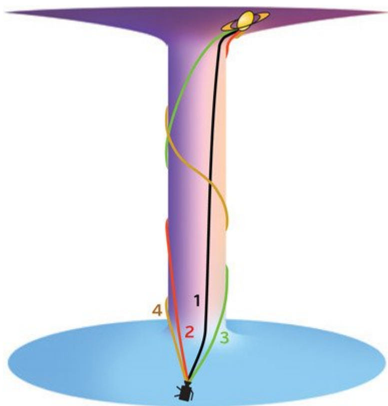
Рис. 15.3. Лучи света, идущие от Сатурна в камеру через червоточину
