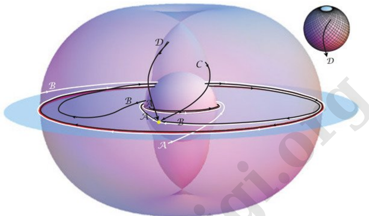
Рис. 8.2. Гаргантюа (центральный сфероид), ее экваториальная плоскость (изображена голубым), ее огненная оболочка (изображена фиолетовым); черными и белыми линиями обозначены лучи света, формирующие для наблюдателя край тени и тонкое кольцо вокруг нее
