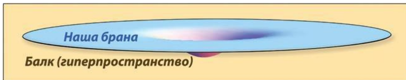
Рис. 3.5. Наша Вселенная в окрестности Солнца, изображенная как двумерная поверхность (или брана), находящаяся в трехмерном балке. В действительности наша брана обладает тремя пространственными измерениями, а балк — четырьмя. Эта схема будет рассмотрена подробнее в главе 4, см. в особенности рис. 4.4
