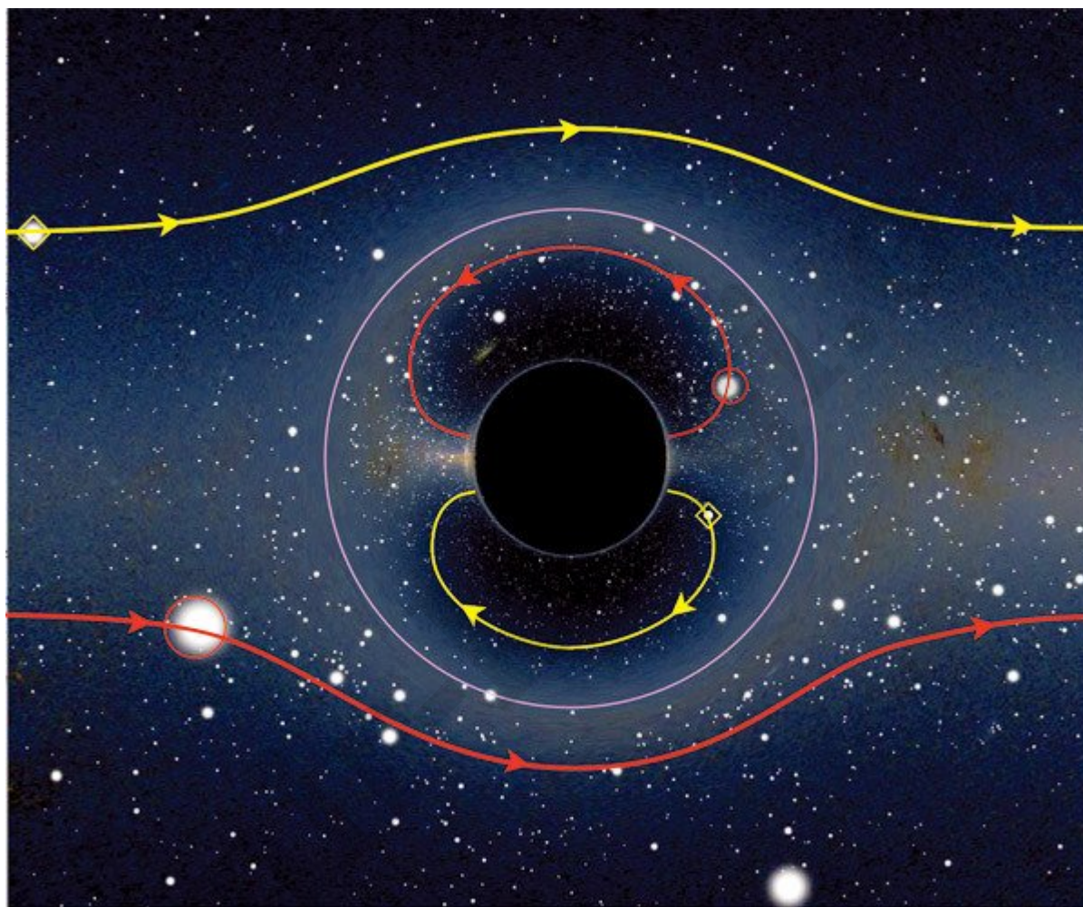
Рис. 8.4. Меняющийся звездный узор, видимый камере при ее движении слева направо по орбите, показанной на рис. 8.3 (Моделирование Алена Риасуэло, см. www2.iap.fr/users/riazuelo/-interstellar .)
