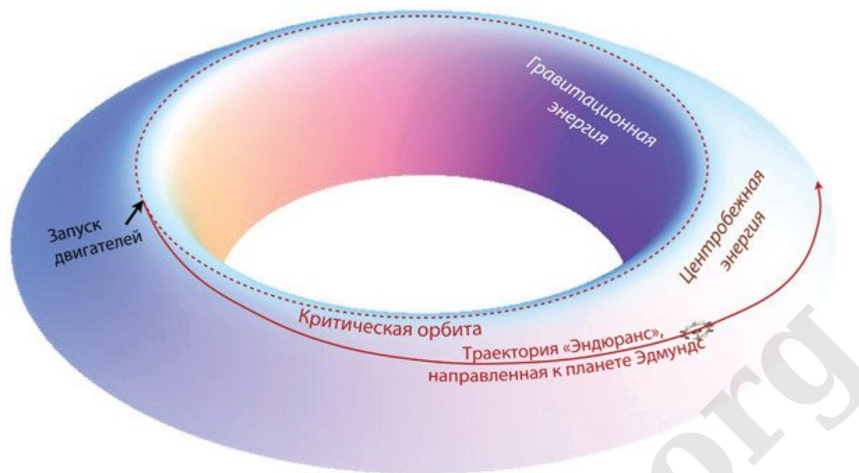
Рис. 27.9. Траектория «Эндюранс», уходящего с критической орбиты по направлению к планете Эдмундс (Изображение «Эндюранс» взято из фильма.)
