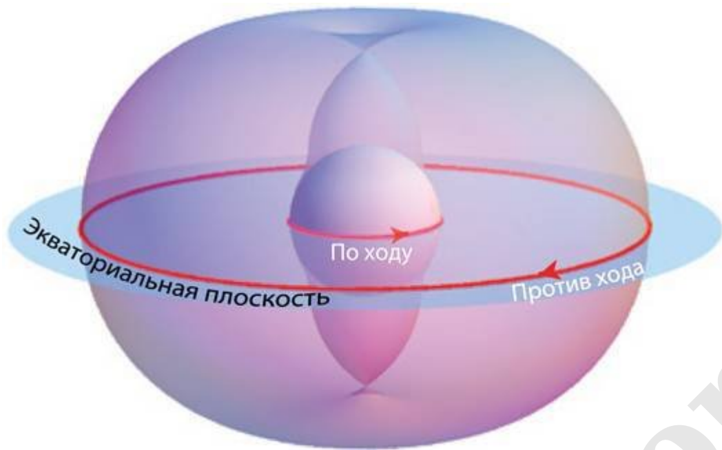
Рис. 6.4. Пончиковобразная область вокруг Гаргантюа, занятая огненной оболочкой
