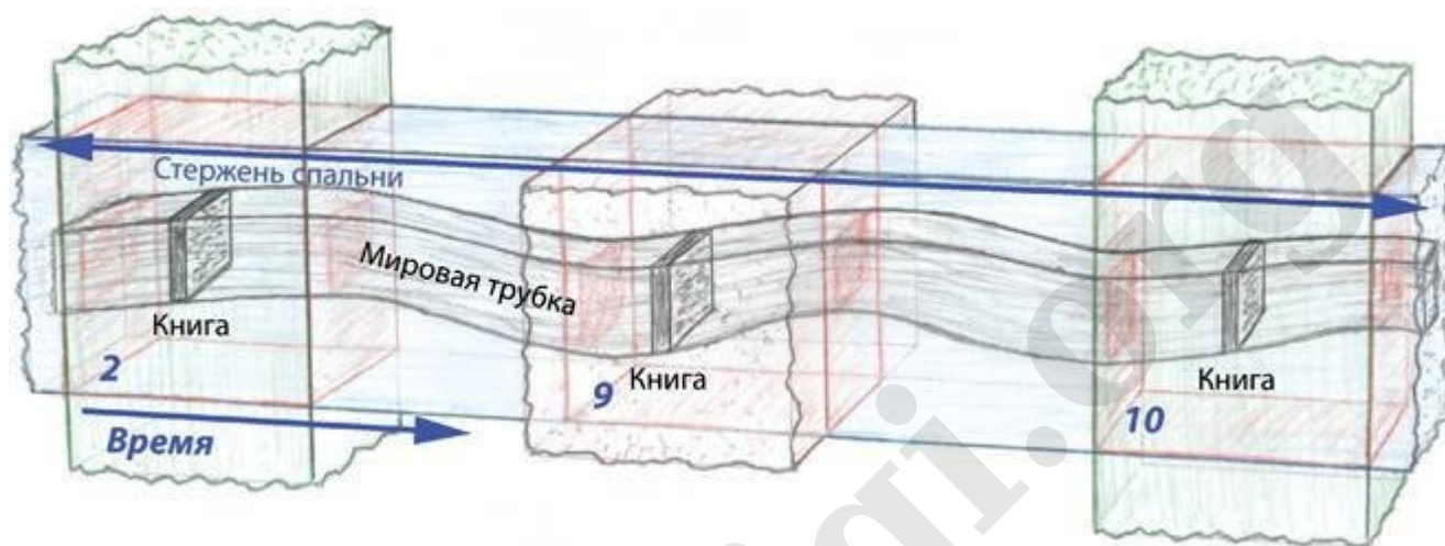
Рис. 30.2. Мировая трубка книги в стержне спальни Мёрф. Книга и мировая трубка на рисунке гораздо больше, чем должны быть в действительности (Мой набросок от руки.)
