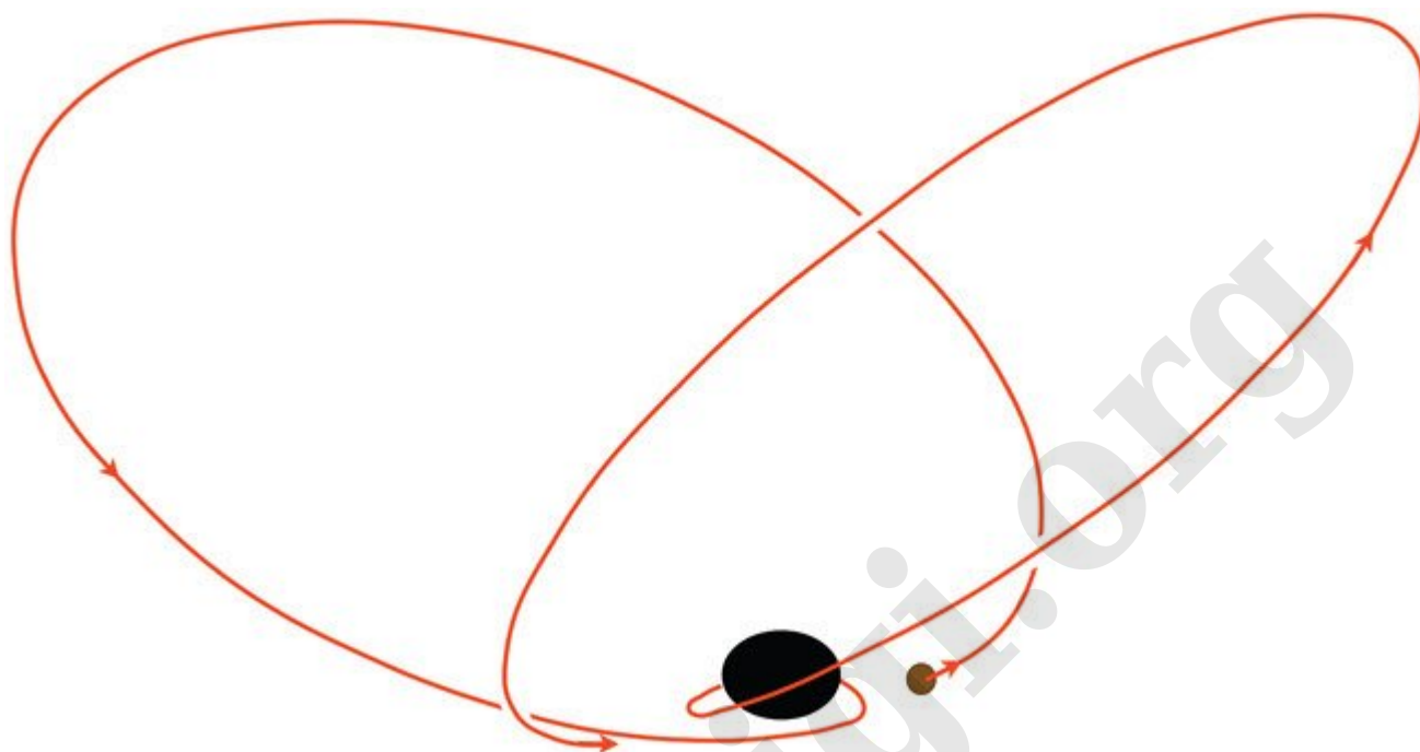
Рис. 19.1. Возможная орбита планеты Манн, вычисленная с помощью крайне дружелюбной интернет-программы, написанной Дэвидом Сароффом, см. demonstrations.wolfram.com/3DKerr-BlackHoleOrbits
