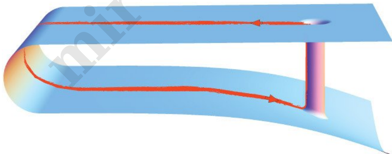
Рис. 30.4. Квантовые флуктуации света, путешествуя по красному пути, нарастают, приводя к взрыву в тот момент, когда червоточина становится машиной времени
