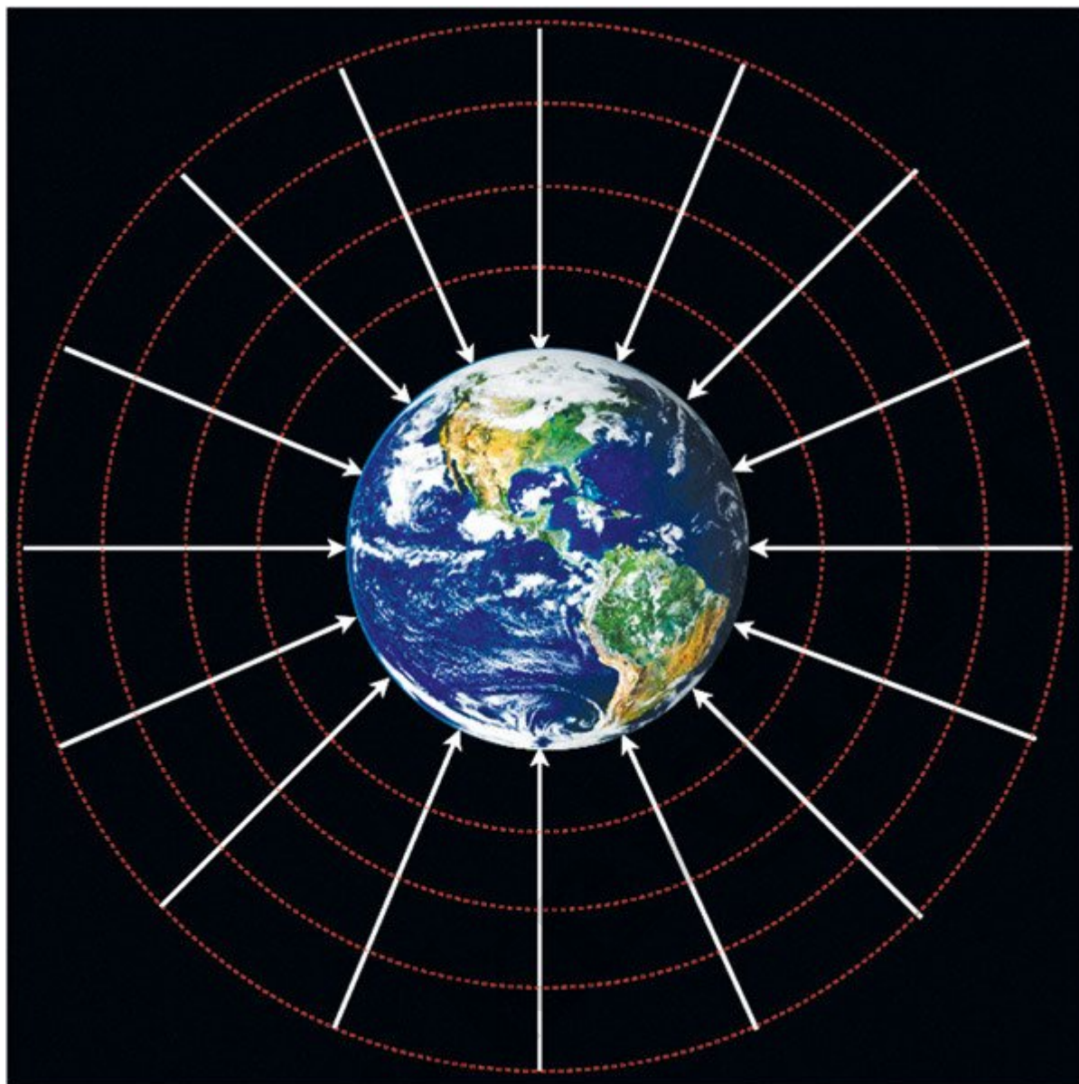
Рис. 2.11. Силовые линии гравитационного поля Земли
