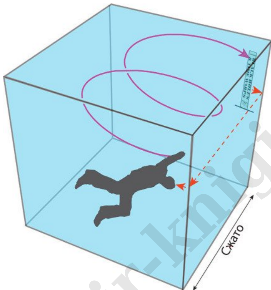
Рис. 30.5. Купер видит книгу, в частности, благодаря лучу света (красный пунктир) и воздействует на книгу с помощью гравитационного сигнала, который распространяется вдоль фиолетовой кривой. Одно из пространственных измерений браны здесь опущено
