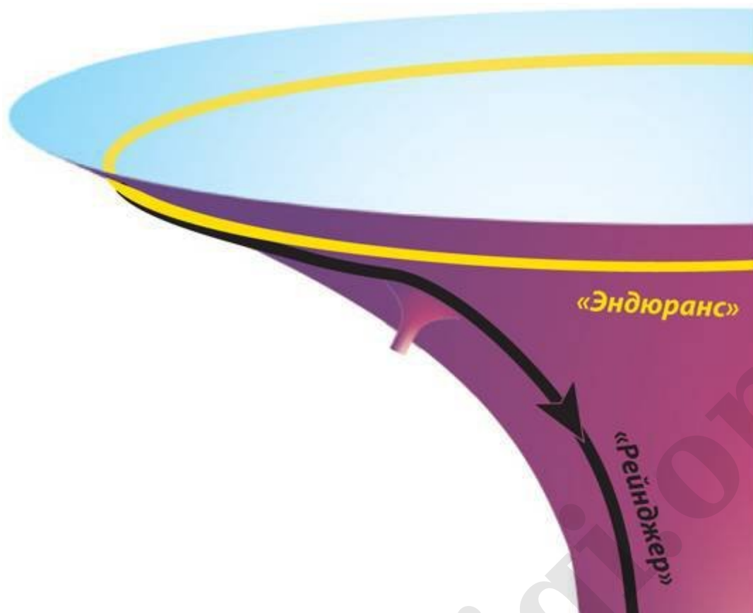
Рис. 7.2. «Рейнджер» выполняет гравитационный маневр вокруг небольшой черной дыры, которая отклоняет его к планете Миллер
